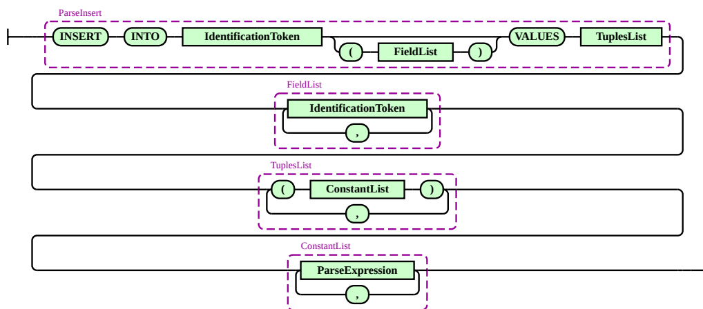
Slika 13: Gramatika ParseInsert sintaktičke kategorije
