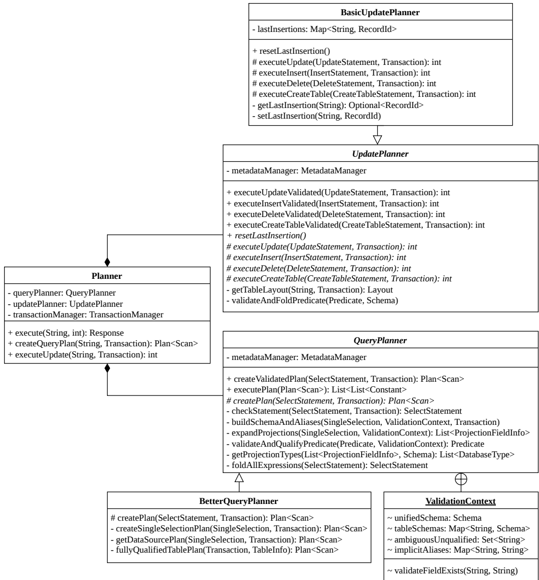
Slika 20: Struktura planera
