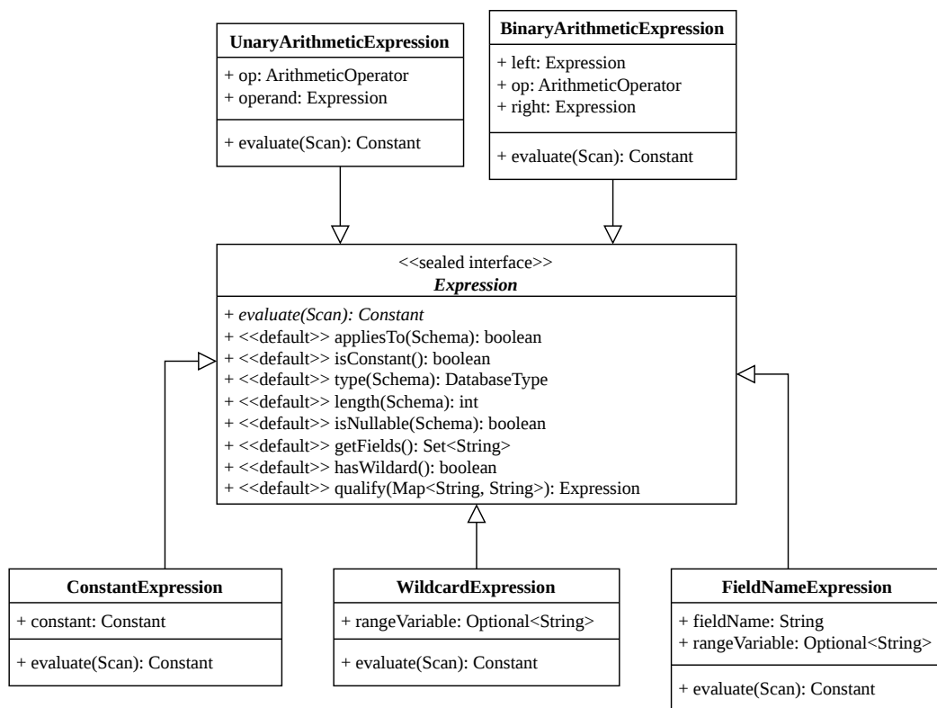
Slika 6: Hijerarhija izraza
