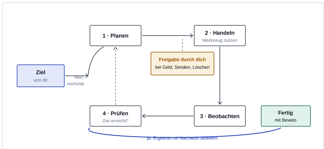
Skizze 4 Der Agenten-Kreislauf. Der Agent plant, handelt, beobachtet und prüft, bis das Ziel erreicht ist. Vor riskanten Schritten muss ein Mensch zustimmen.
