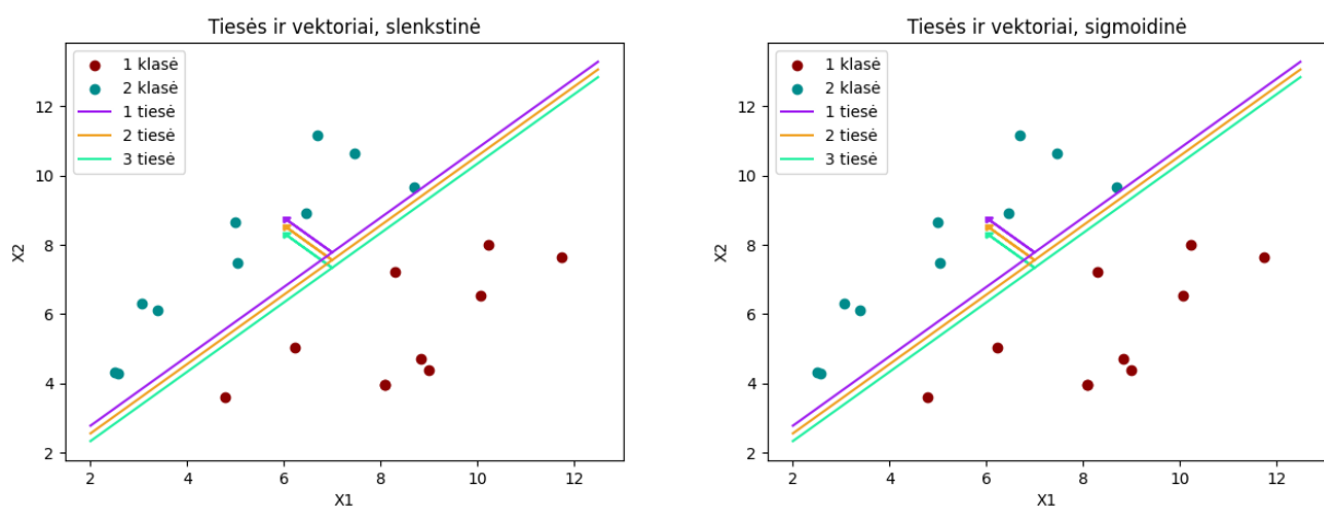
(a) Tiesės gautos su slenkstine aktyvacijos funkcija (b) Tiesės gautos su sigmoidine aktyvacijos funkcija
