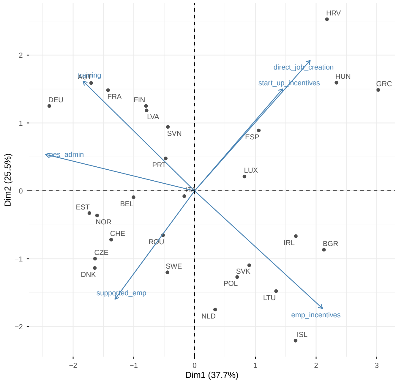
PCA biplot – ALMP policy mix
