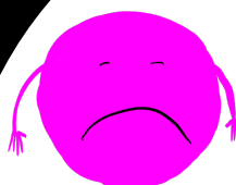
Elektron
