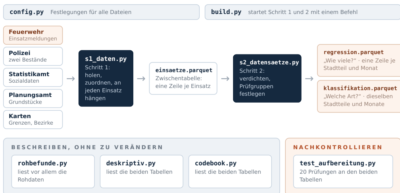
Abbildung 1: Der Weg der Daten durch den Ordner. Nur s1_daten.py und s2_datensaetze.py erzeugen Daten. Die drei Dateien in der linken unteren Leiste lesen nur und legen ihre Befunde in results/ ab. Die Prüfdatei aus tests/ kontrolliert die beiden fertigen Tabellen.
