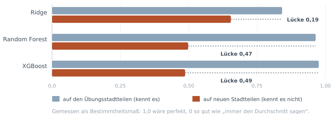
Abbildung 17: Werte aus Abschnitt 6.1 und Tabelle 9 der Arbeit. Alle drei Verfahren verlieren beim Sprung auf unbekannte Stadtteile — die beiden Baumverfahren aber rund zweieinhalbmals so viel wie Ridge.
