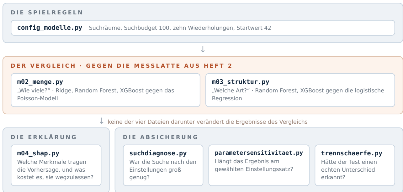
Abbildung 1: Der Kern des Ordners sind die beiden Vergleichsdateien, für jede Frage der Arbeit eine. Von den vier Dateien darunter erklärt eine die Ergebnisse, drei prüfen, wie belastbar sie sind.
