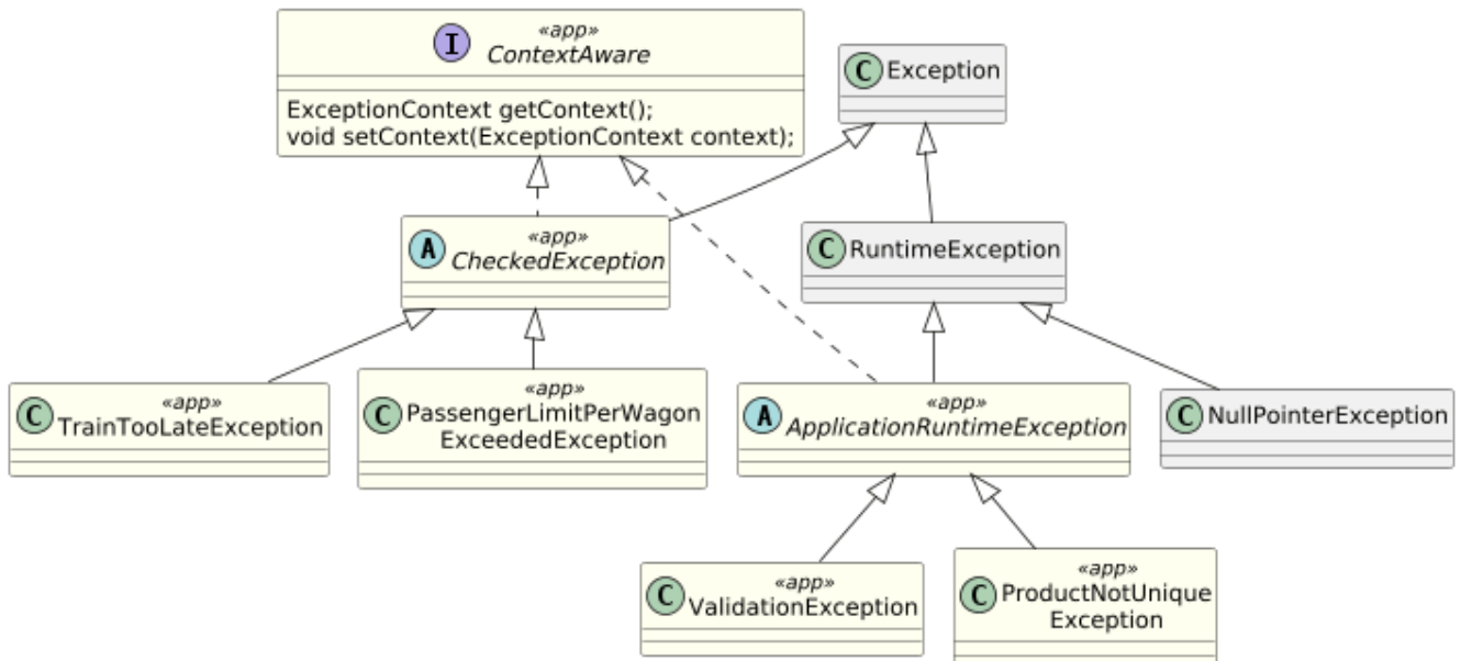
Figure 2. Exceptions Beispiel
