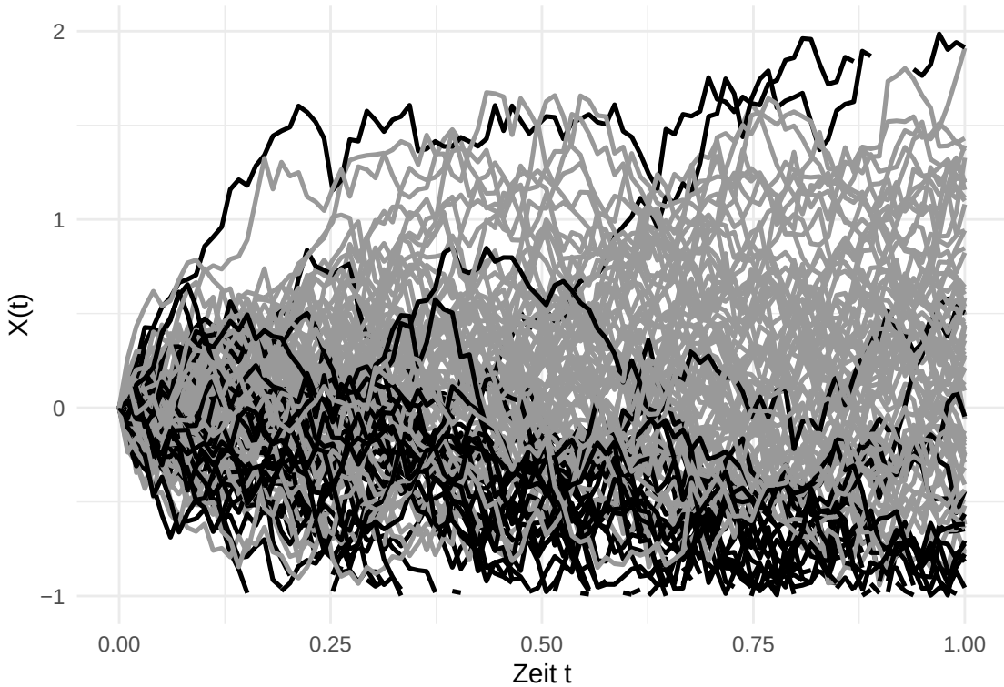
Brownian-Pfade nach MNAR-Zensur
