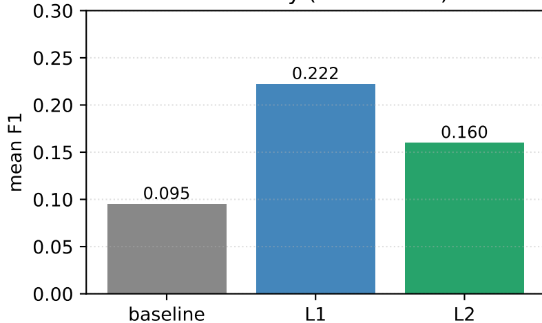
CUAD-only (5 contracts)
