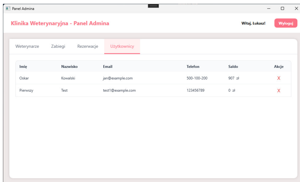
Rys. 5.53. Widok zakładki Użytkownicy w panelu administratora.
