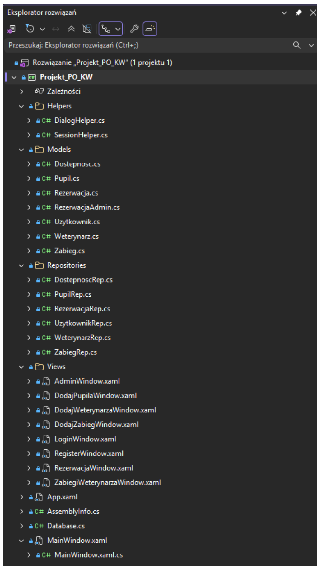
Rys. 3.2. Struktura klas w projekcie.
