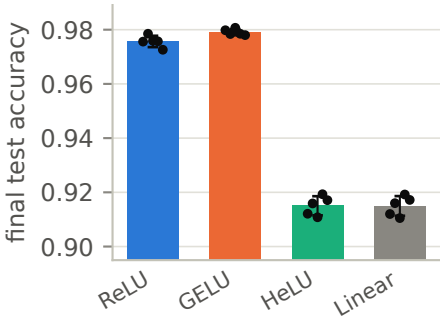
MNIST MLP
