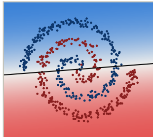
Identity · acc 0.649
