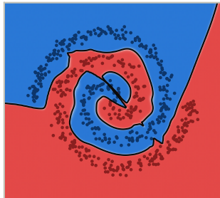
GELU · acc 0.996
