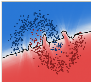
HeLU · acc 0.630
