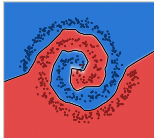
ReLU · acc 0.996
