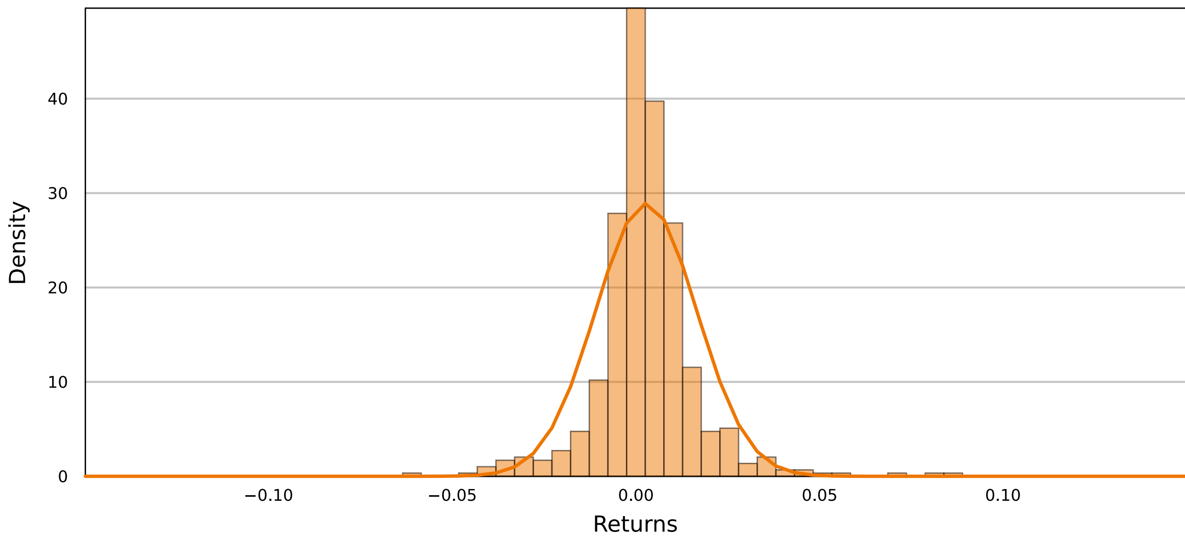
SSE 50 Index
