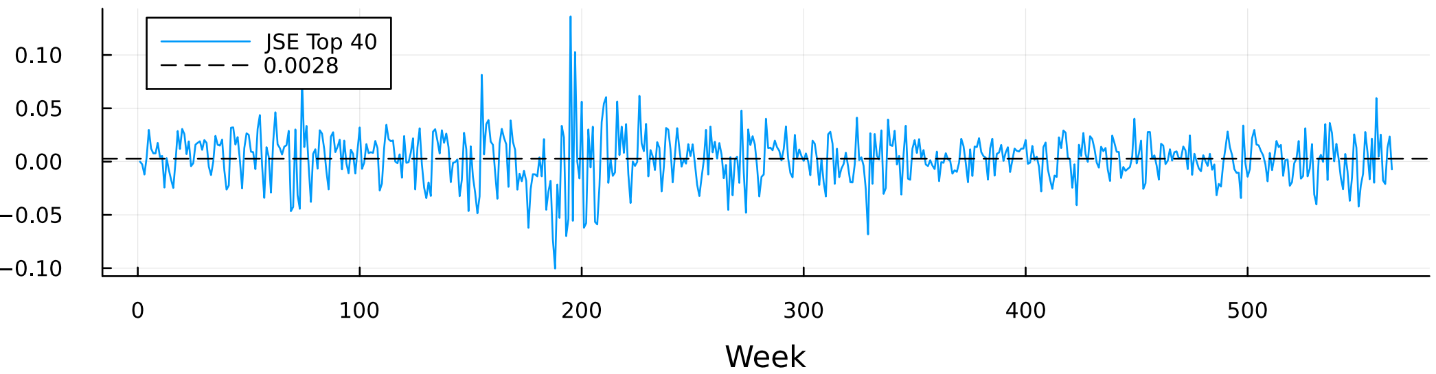
JSE Top 40 Index
