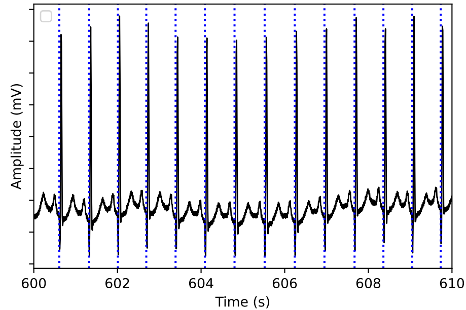
Electrocardiogram: a13
