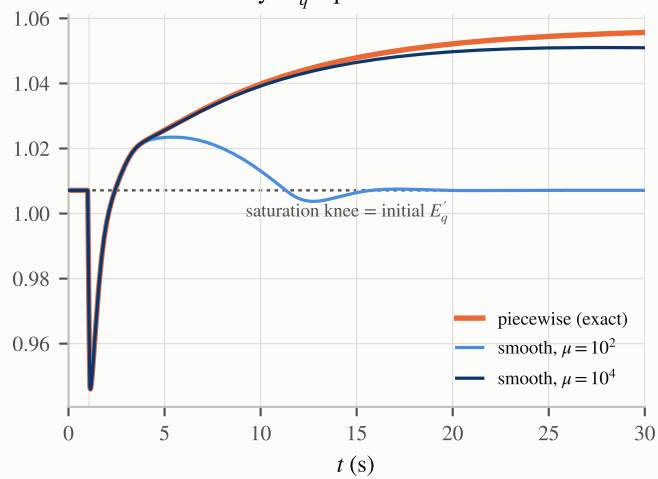
GENSAL boundary: E'_q equilibrium shift
