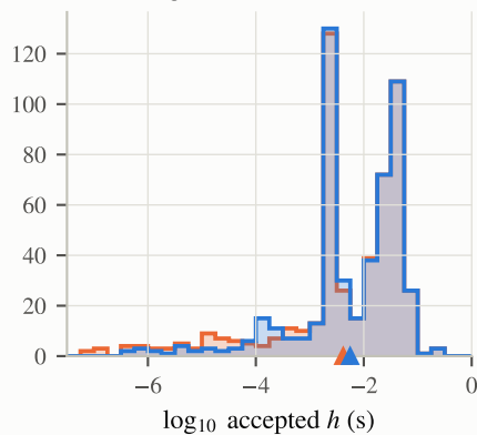
ACTIVSg500
