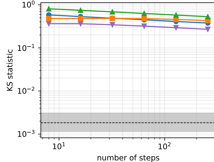
Regime E
