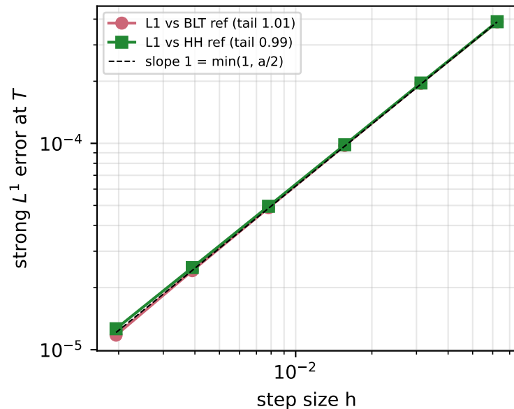
Regime A: a = \delta = 16
