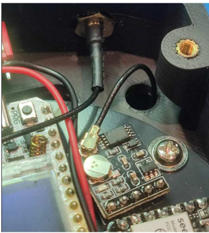
GPS Antenna
