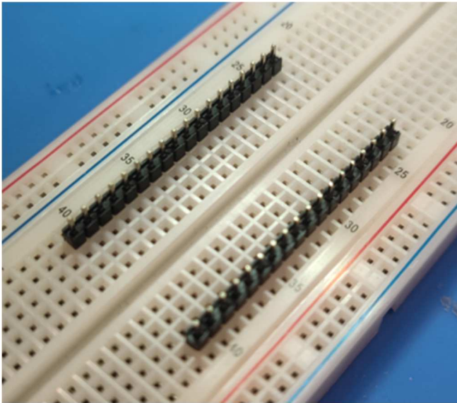
ESP module
