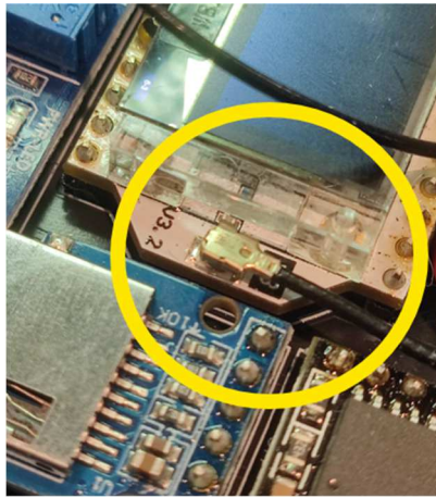
LORA Antenna
