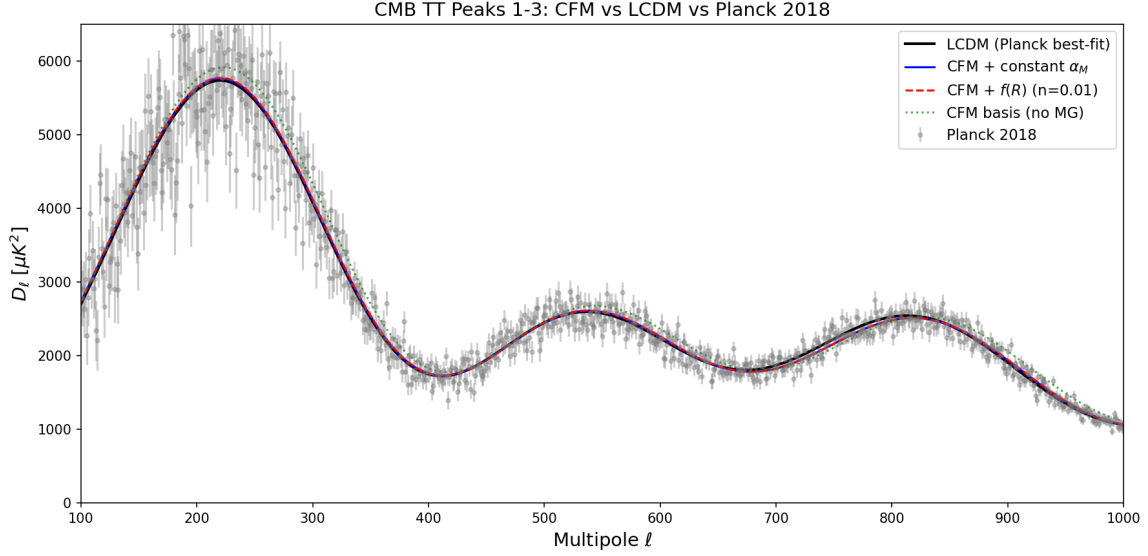
Abbildung 2: Detailansicht der ersten drei akustischen Peaks. Die cfm_fR-Modifikation verschiebt die Position des ersten Peaks durch den frühen ISW-Effekt (gesteuert durch \alpha_M ), ohne die akustische Winkelskala \theta_s zu ändern. Das Verhältnis dritter-zu-erster Peak bleibt erhalten.
