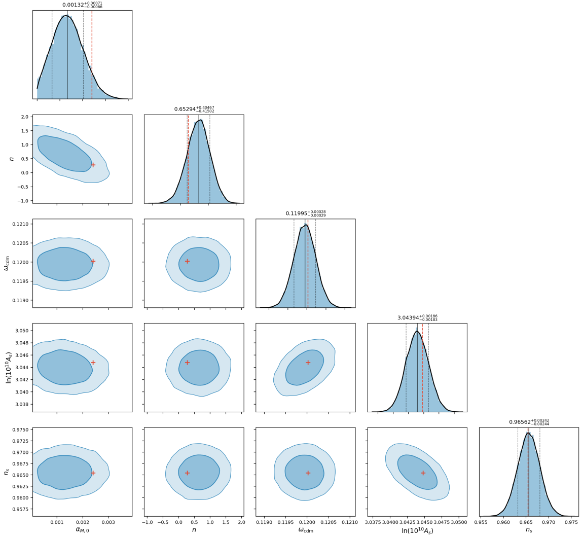
Abbildung 3: Corner-Plot der cfm_fr-MCMC-Posterior (240.000 Samples von 48 Walkern, 5.000 Produktionsschritte). Diagonale Panels zeigen die marginalisierten 1D-Posteriorien mit 68%-Kreditätsintervallen (gestrichelte Linien). Off-diagonale Panels zeigen 2D-Konturen bei 68% und 95% Kreditätsniveau mit gefüllten Bereichen. Rote Kreuze markieren den Best-Fit-Punkt ( \chi^2 = 6625,1 , \Delta\chi^2 = -3,7 vs. \Lambda\text{CDM} ). Die Anti-Korrelation \rho(\alpha_{M,0}, n) = -0,61 ist deutlich sichtbar, während alle Kreuzkorrelationen zwischen MG- und Standardparametern |\rho| < 0,08 erfüllen.
