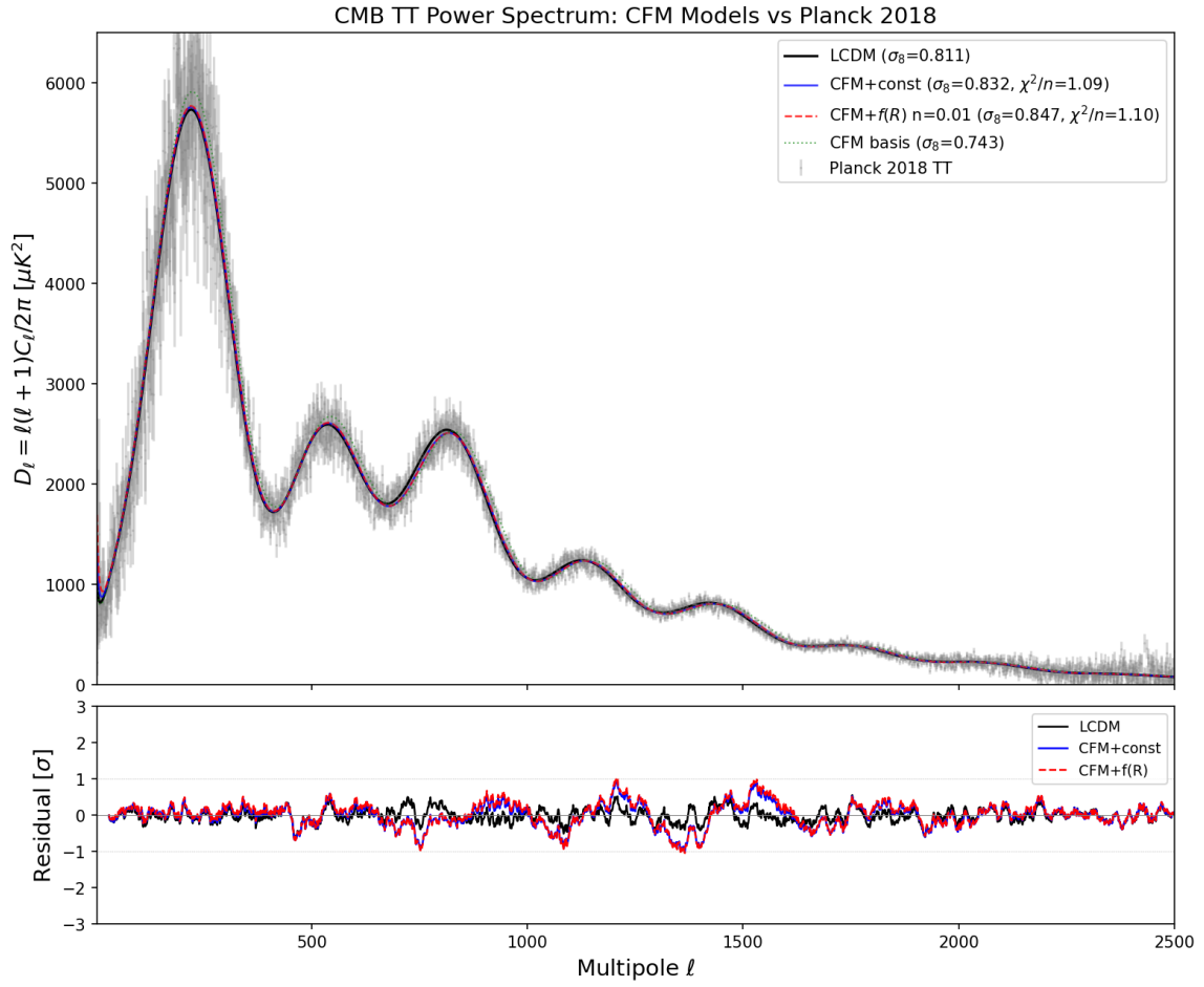
Abbildung 1: CMB-Temperatur-Leistungsspektrum \mathcal{D}_\ell^{TT} für \Lambda CDM (schwarz) und cfm_fR-Modelle mit verschiedenen \alpha_{M,0} -Werten (farbig), verglichen mit Planck-2018-Daten (graue Punkte mit Fehlerbalken). Alle CRM-Modelle sind durch volle Boltzmann-Integration in hi_class v2.9.4 berechnet. Das Residuenpanel zeigt \Delta\mathcal{D}_\ell/\sigma_\ell relativ zu Planck. Die CRM-Modifikation verstärkt die Leistung bei niedrigen Multipolen ( \ell \lesssim 200 ) durch den frühen integrierten Sachs-Wolfe-Effekt.
