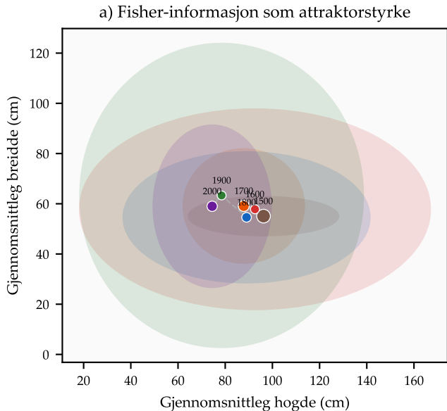
Fig. 5: Informasjonsgeometrisk overflate
