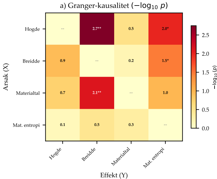
Fig. 5: Granger-kausaltet -- kva driv formending?
