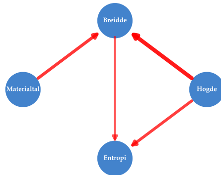
b) Kausale pilar ( p < 0.05 )
