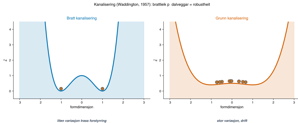
Figur 4. Kanalisering etter Waddington (1957): brattleiken på dalveggane gjev robustheit mot forstyring. Venstre: bratte kanalar held realiserte former nær eit lokalt optimum trass i varierende initialtilstand og påverknad. Høgre: grunne kanalar gjev drift og stor formvariasjon. Kanalisering er målbar og kan estimerast empirisk frå formdata.
