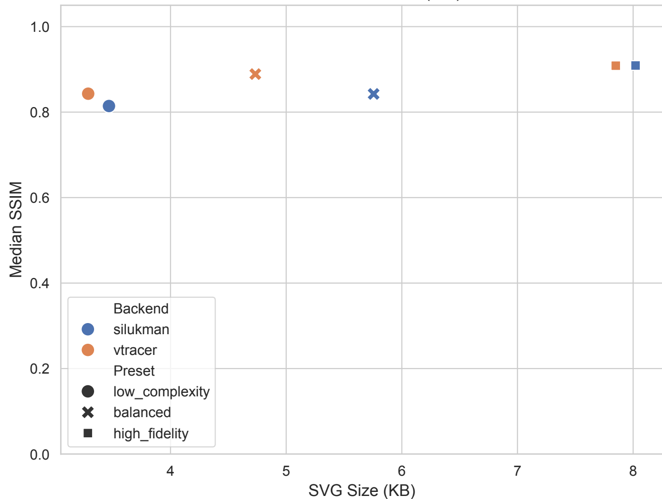
SSIM vs SVG Size (KB)
