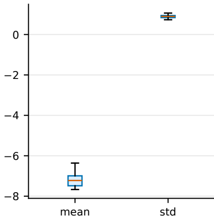
cls logits
