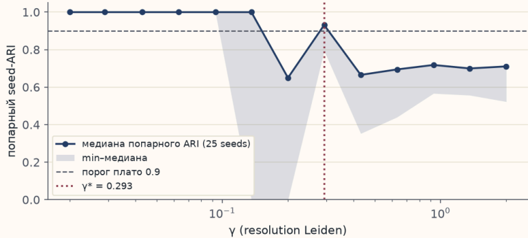
F1. Плато-правило: стабилен только макро-уровень k=3 попарный ARI между 25 seed-прогонами Leiden против resolution \gamma
