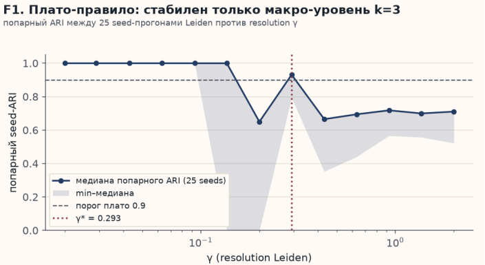
ГЕЙТ УСТОЙЧИВОСТИ: СОВПАДЕНИЕ РАЗБИЕНИЙ (ARI) ПРИ 25 ПЕРЕЗАПУСКАХ ПО СИЛЕ ДЕТАЛИЗАЦИИ \gamma
