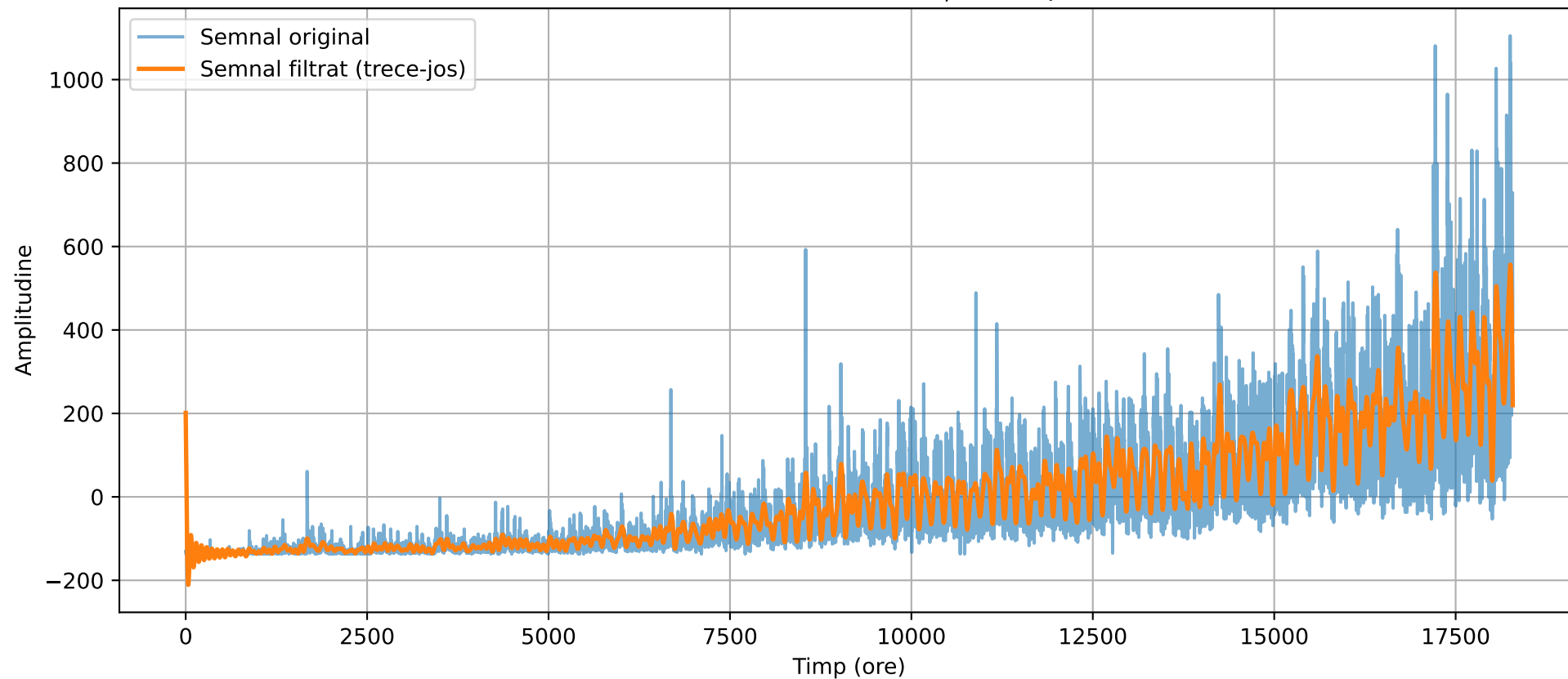
Filtrare în domeniul frecvenței (low-pass)
