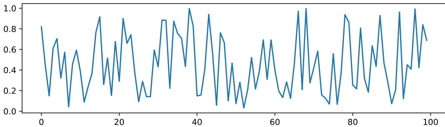
x[n]*x[n]
