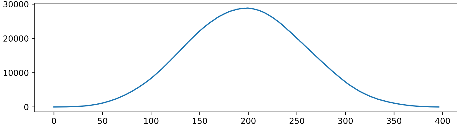
x[n]*x[n]*x[n]*x[n]
