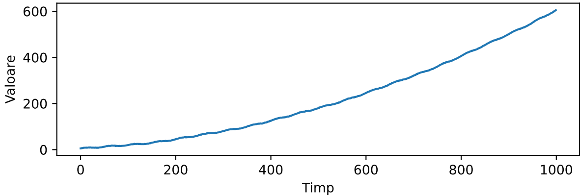
Mediere exponentiala dubla
