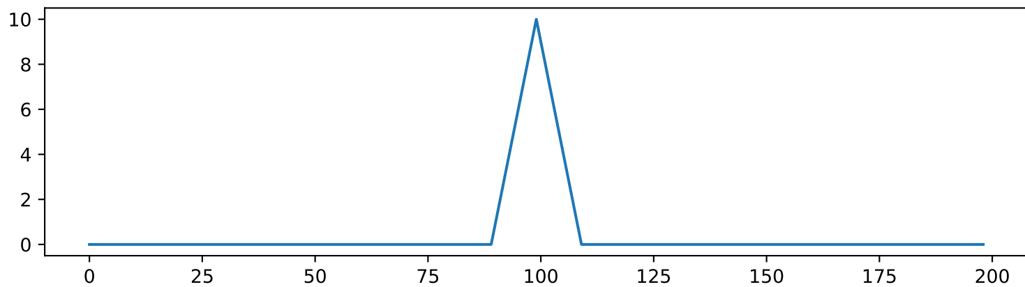
x[n]*x[n]*x[n]
