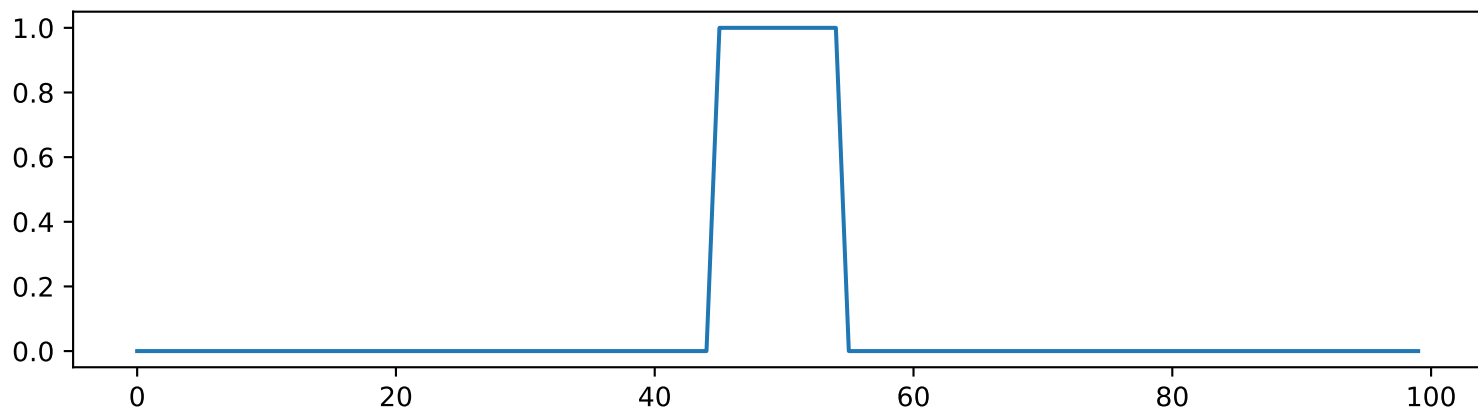
x[n]*x[n]
