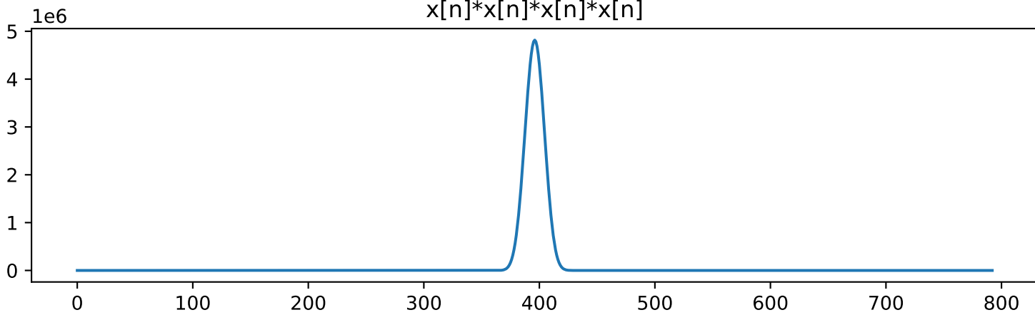
x[n]*x[n]*x[n]*x[n]
