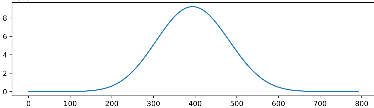
x[n]*x[n]*x[n]*x[n]
