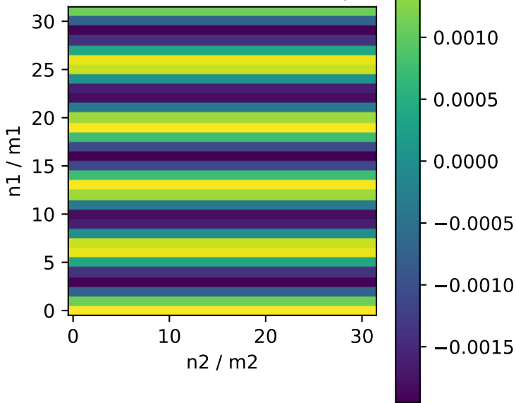
IDFT(Y4)-domeniul timp
