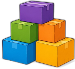
boxes
