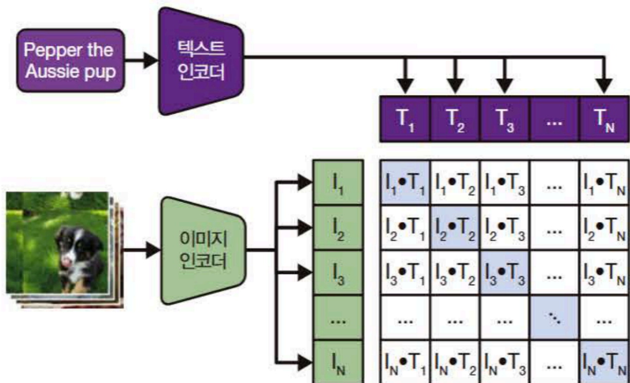
그림 16. 『핸즈온 생성형 AI』 136쪽 그림 3-7 원본 발췌. 초록색 행은 이미지, 보라색 열은 문장이다. 대각선은 함께 주어진 올바른 짝이다. 이 그림은 OpenAI CLIP 구조를 참고한 교재 도식이다.
