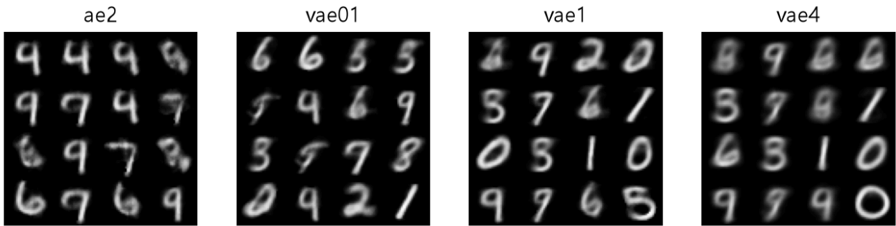
그림 15. 같은 seed로 뽑은 동일한 표준정규 좌표를 사용했다. VAE는 이 prior와 연결하도록 학습하지만, AE는 그런 제약이 없다. 표본 16개의 인상만으로 생성 분포 전체의 품질을 평가하지 않는다. 숫자가 불분명하거나 서로 비슷한 결과도 관찰 내용으로 남긴다.
