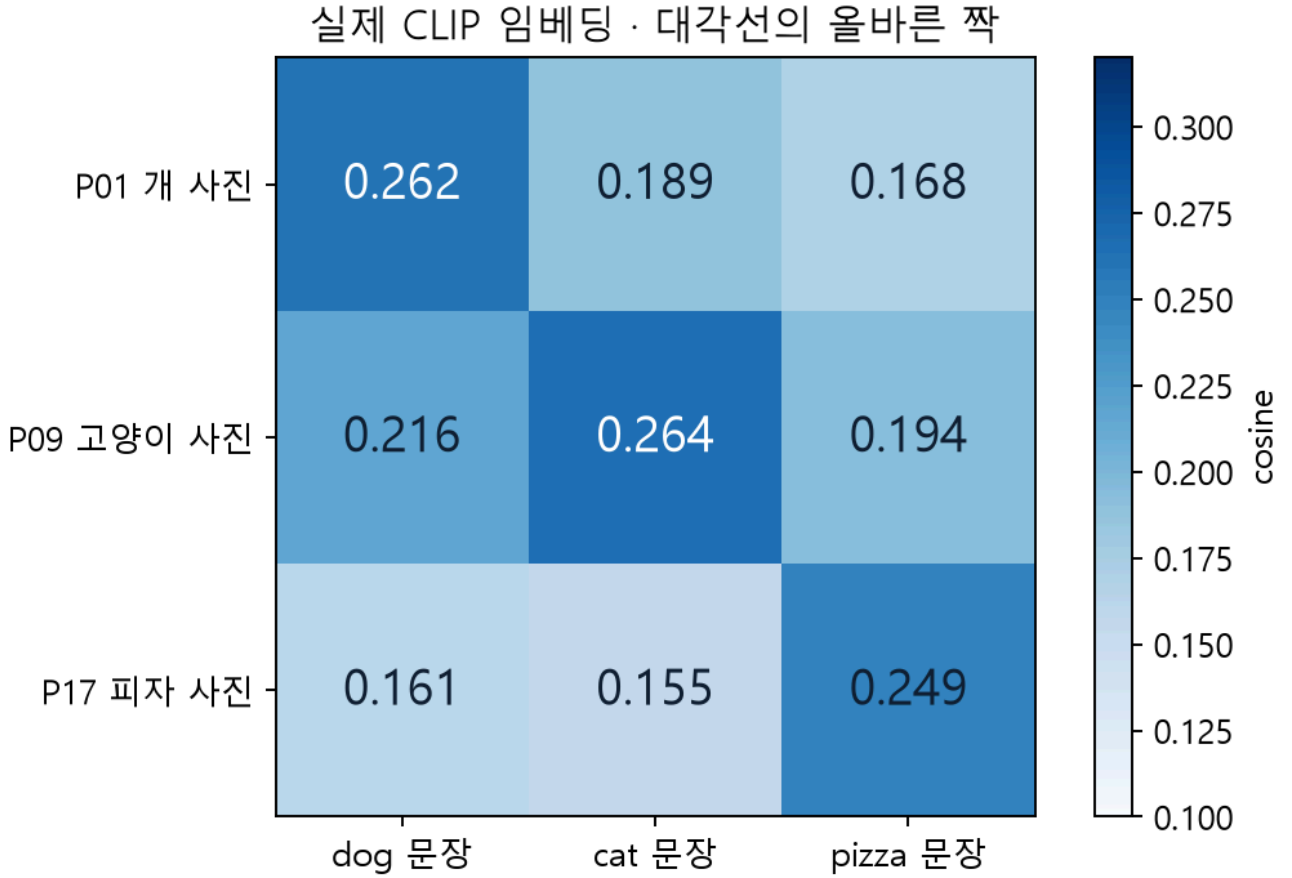
그림 18. P01 개, P09 고양이, P17 피자 사진의 실제 유사도. 대각선이 해당 행·열의 다른 후보보다 큰지 읽는다. 이 3쌍에서의 성공이 모든 장면에서의 정확도를 뜻하지 않는다.
