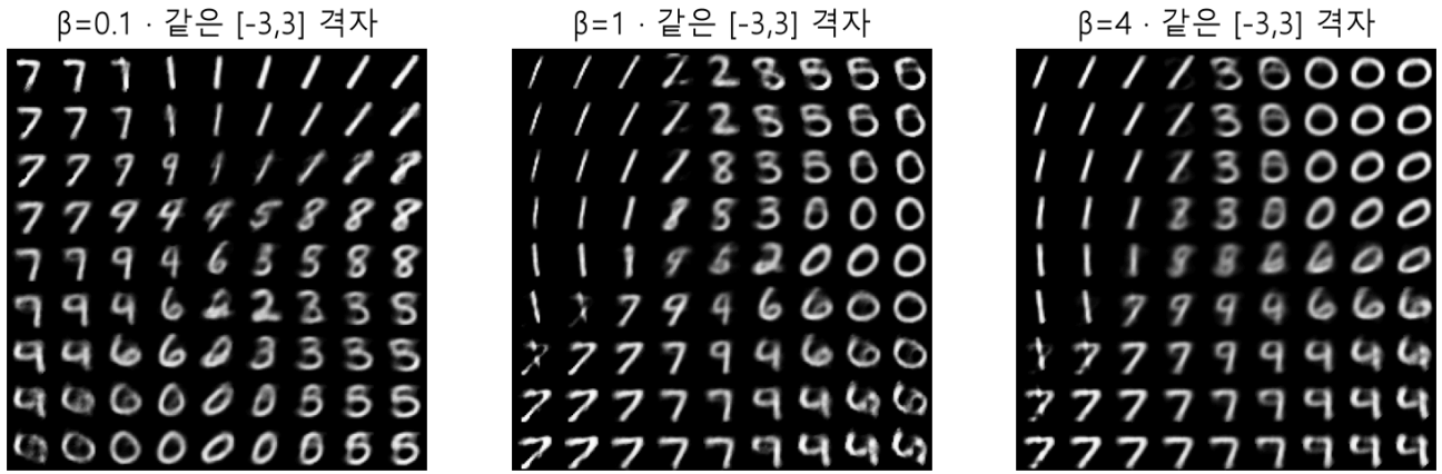
그림 12. 같은 2차원 격자 [-3,3] \times [-3,3] 를 세 모델에서 디코딩했다. 모델을 세 번 따로 학습한 비교다. 화면의 모델 선택은 체크포인트 전환이며, 슬라이더가 즉시 재학습하는 것처럼 해석하지 않는다. 격자는 균일한 좌표 배치이고 정규분포 샘플이 아니다.
