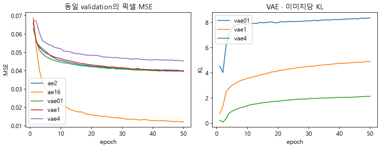
그림 11. 수업용 작은 모델의 실측. 왼쪽은 epoch 끝 모델의 validation MSE, 오른쪽은 해당 epoch의 학습 배치 KL 평균이다. 오른쪽은 갱신 중인 여러 상태의 평균이므로 왼쪽과 측정 방식도 다르다.
