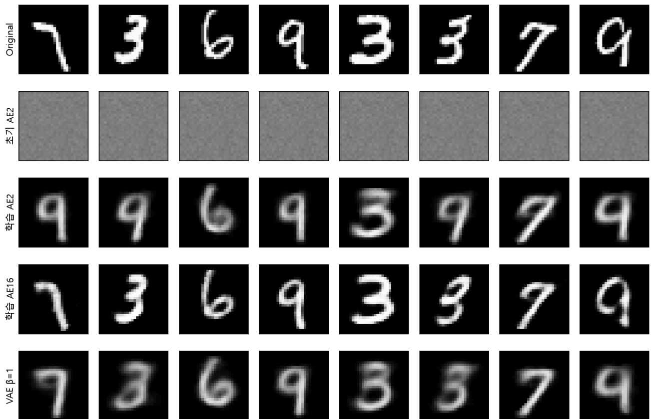
그림 4. 수업 코드의 실제 실행. 테스트의 첫 8장을 고정 순서로 사용했다. 잘 복원된 그림만 고른 결과가 아니다. 모든 행의 밝기 범위는 0~1이다. 획의 위치·두께·굵어짐을 세로로 비교한다.
