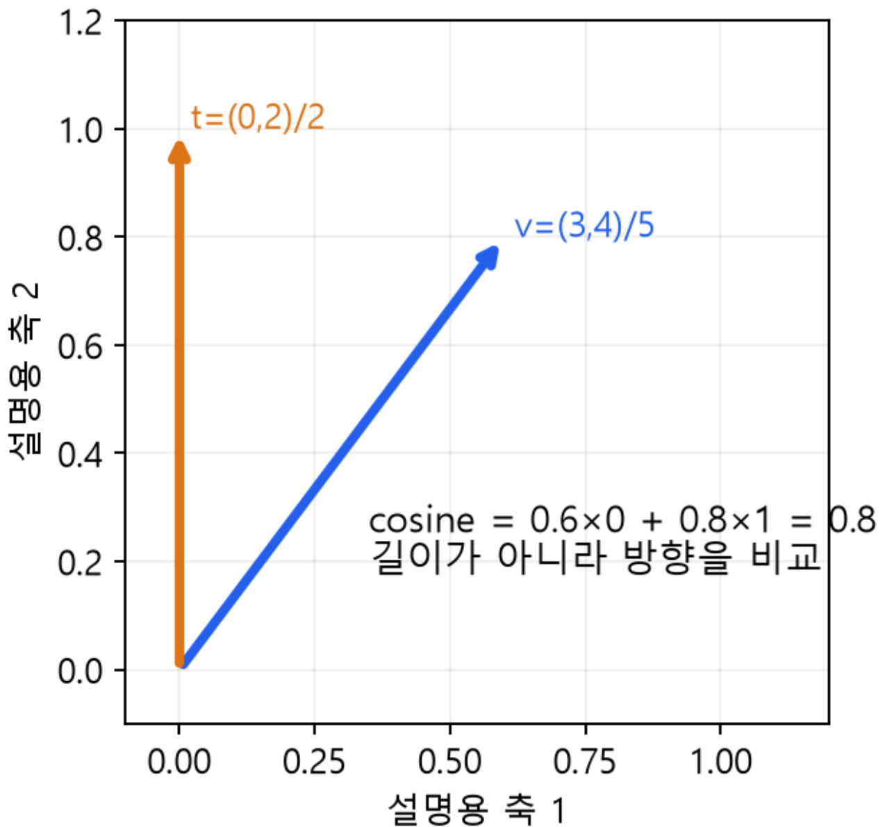
그림 17. 설명용 2차원 예. (3, 4) 의 길이는 5, (0, 2) 의 길이는 2이므로 정규화하면 (0.6, 0.8) 과 (0, 1) 이다. 코사인은 0.8이다. 실제 CLIP은 이 그림의 두 축이 아니라 512차원을 사용한다.
