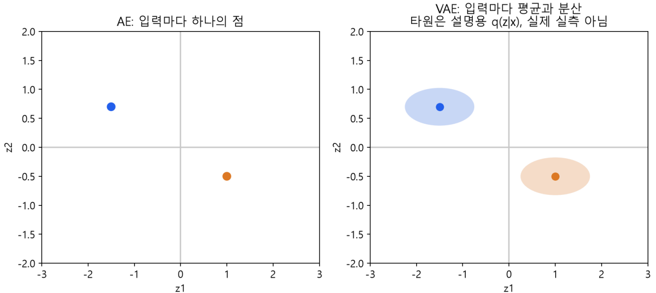
그림 8. 분포의 필요성을 설명하는 자체 도식이며 실측 산점도가 아니다. 타원의 중심은 평균, 축 방향의 폭은 표준편차와 연결된다. 대각 공분산은 좌표 사이 공분산을 0으로 두는 가정이며, 모든 좌표의 분산이 같다는 가정이 아니다.
