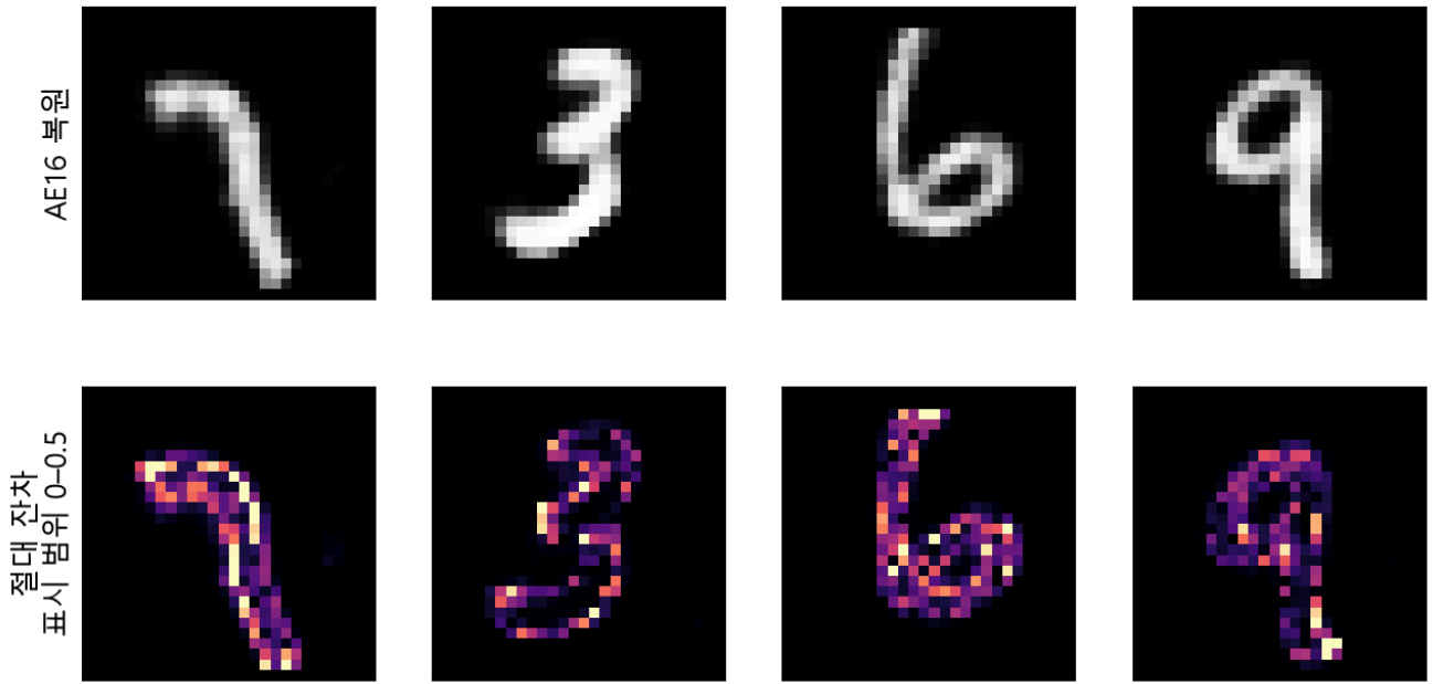
그림 5. 잔차는 |x - \hat{x}| 다. 그림에서는 위치를 보기 쉽게 표시 범위를 0-0.5로 고정했고, 웹 앱은 0-1로 고정한다. 밝은 부분은 차이가 큰 픽셀이다. 이미지마다 자동으로 밝기를 늘리면 서로 다른 오차 크기를 잘못 비교할 수 있다.
