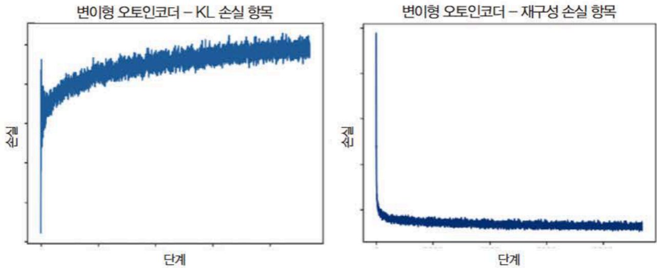
그림 10. 『핸즈온 생성형 AI』 129쪽 그림 3-5 원본 발췌. 교재에서 관찰한 학습 곡선이다. KL이 모든 단계에서 감소해야 정상인 것은 아니다. 복원에 유용한 정보를 더 담으며 KL이 증가할 수도 있다. 이 그림을 아래 수업 실행의 측정 결과와 섞지 않는다.
