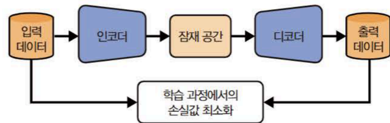
그림 2. 『핸즈온 생성형 AI』 97쪽 그림 3-2 원본 발체. 위쪽 화살표는 순전파, 아래쪽 연결은 입력과 출력의 비교로 읽는다. 아래 화살표가 이미지를 다시 인코더에 넣는 별도 생성 과정이라는 뜻은 아니다.
