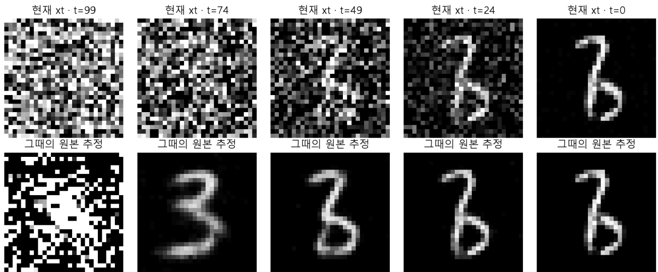
그림 4. 기존 4000회 학습 체크포인트, seed42, DDPM 100회 갱신의 실제 출력. 위 행은 모델에 들어간 현재 상태, 아래 행은 그 시점의 원본 추정이다. 초기 원본 추정이 애매할 수 있으며, 하단 이미지를 매번 바로 다음 입력으로 넣은 실험이 아니다.
