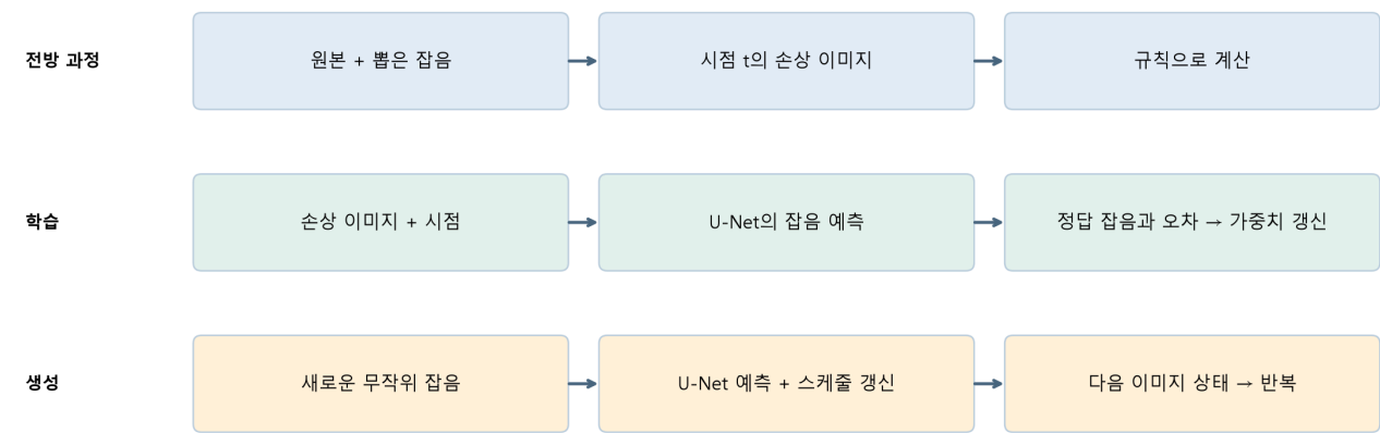
그림 2. 수업용 자체 도식. 파랑은 손상 데이터를 만드는 계산, 초록은 신경망의 가중치를 바꾸는 학습, 주황은 이미지 상태를 바꾸는 생성이다. 같은 U-Net을 반복 호출해도 생성 중에 가중치가 학습되는 것은 아니다.
