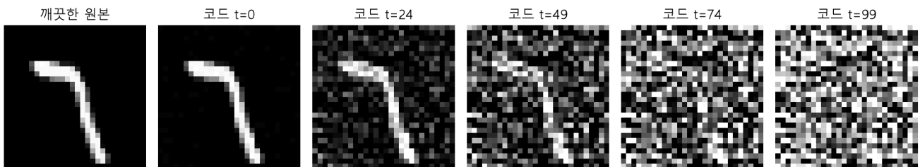
그림 3. 실제 MNIST 테스트 이미지와 seed42의 잡음. 원본과 잡음을 고정하고 시점만 바꾸었다. 이는 각 시점의 주변분포를 비교하는 실험이다. 단계마다 새 잡음을 뽑아 이어 붙이는 하나의 Markov 경로와 구별한다. 표시 범위만 [-1,1]로 고정하며 계산 텐서는 자르지 않는다.
