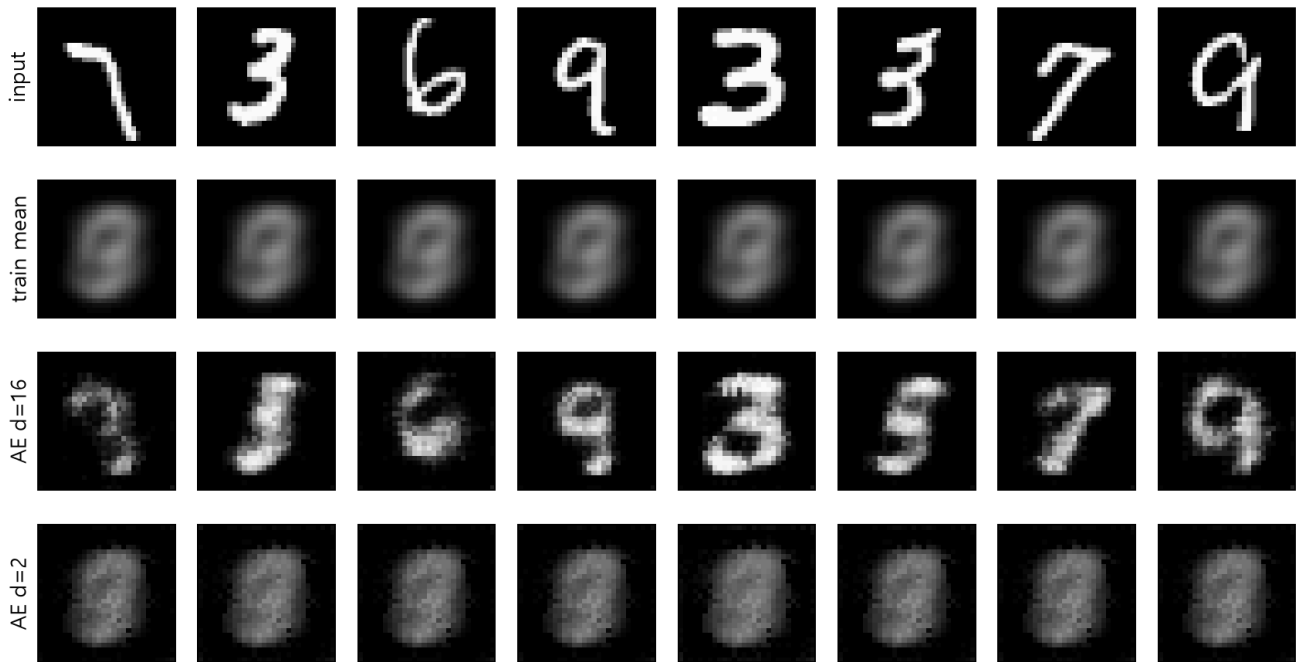
그림7. test의 첫8장을 고정 순서로 표시했다. 잘된 사례만 고른 그림이 아니다. 모든 행은 동일한0-1 밝기 범 위다. MSE와 함께 획이 흐려지거나 서로 붙은 위치를 확인한다.
