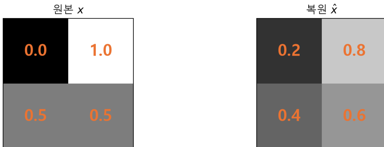
그림5. 자체 작성한 4픽셀 수계산 예. 차이의 제곱은 0.04, 0.04, 0.01, 0.01이고 합은 0.1, 평균은 0.025다.
