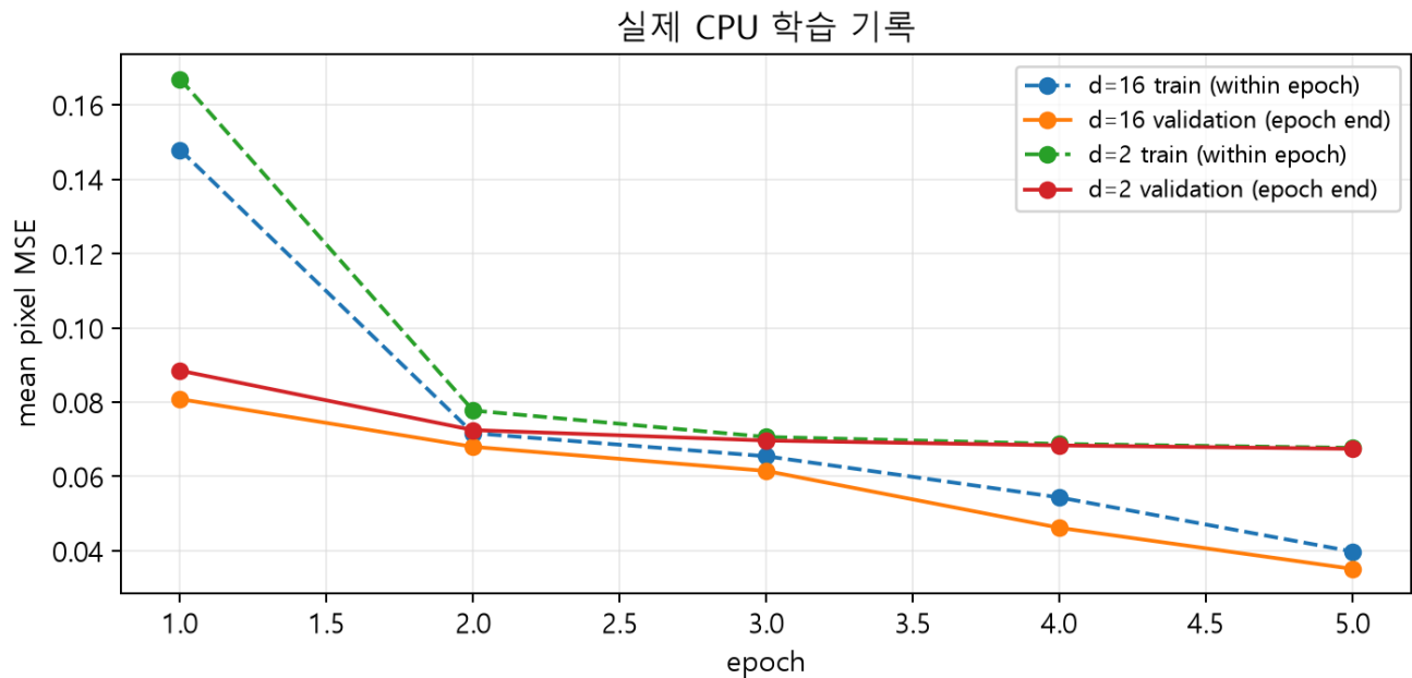
그림6. Python3.12.10·PyTorch2.8 CPU 실측. train선은 epoch 중 갱신되는 모델들의 배치 손실 평균이고 validation선은 epoch 마지막 모델의 평가다. 그래서 두 선의 차이를 전부 일반화 차이라고 단정하지 않는다. 다섯 epoch을 사전에 고정했고 test를 보며 학습 횟수를 선택하지 않았다.
