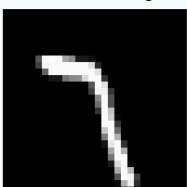
깨끗한 x_0
