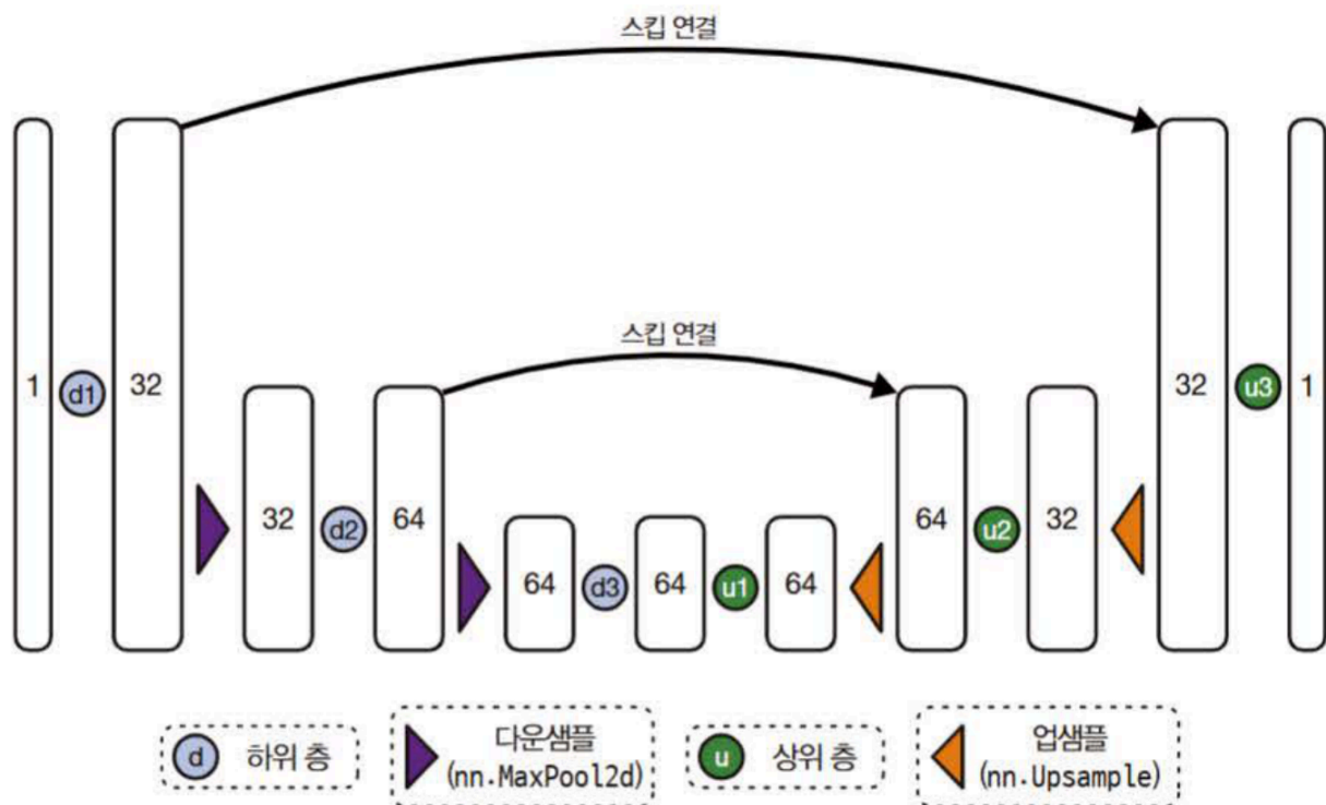
그림 4-3 간단한 U-Net의 구조
