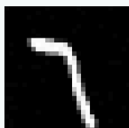
코드 t=0
