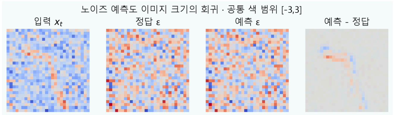
그림 6. 실제 test 한 장, 코드 t49에서 입력·정답 epsilon·학습 모델의 예측·잔차를 표시했다. 네 그림은 공통 색 범위 [-3,3]을 사용한다. 예측 잡음은 숫자 라벨도, 완성된 숫자 이미지도 아니다. 잔차가 남는 위치에서 모델의 예측이 불완전함을 확인한다.
