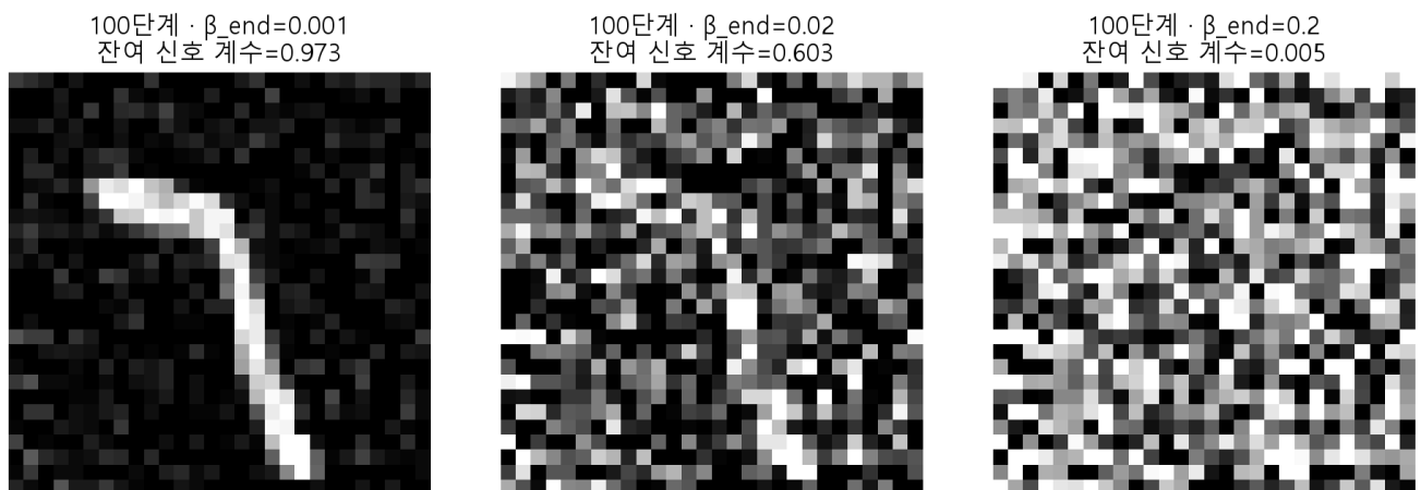
그림 6. 모두 100단계 linear 스케줄이고 beta 시작값은 0.0001이다. 끝값만 바꾸었다. 표시된 수치는 마지막 원본 계수다. 원본과 기본 잡음은 같다. 스케줄을 비교한 전방 실험이며, 세 생성 모델을 따로 학습한 결과가 아니다.
