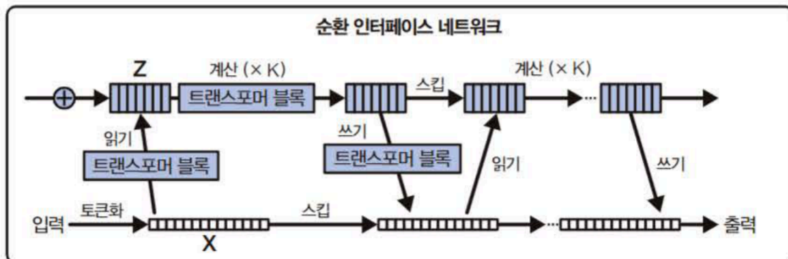
림 4-10 U-Net, UViT, 순환 인터페이스 네트워크의 비교
