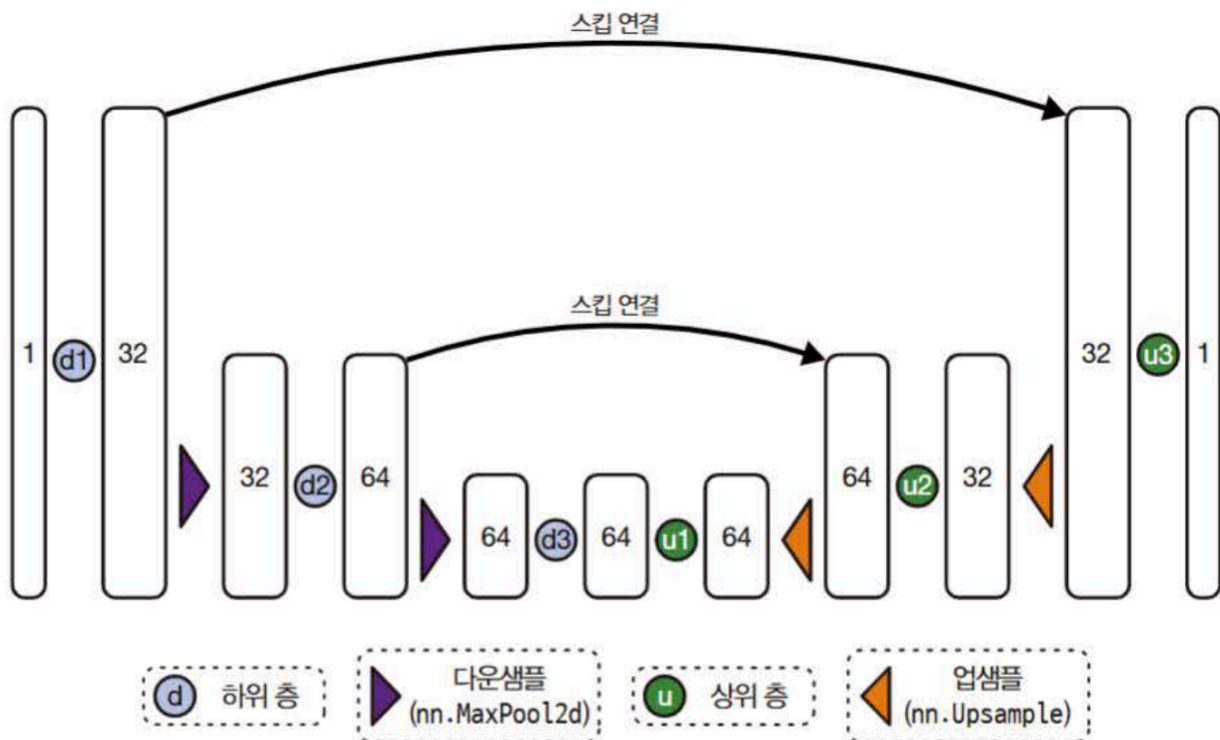
그림 4-7 기본 U-Net의 구조
