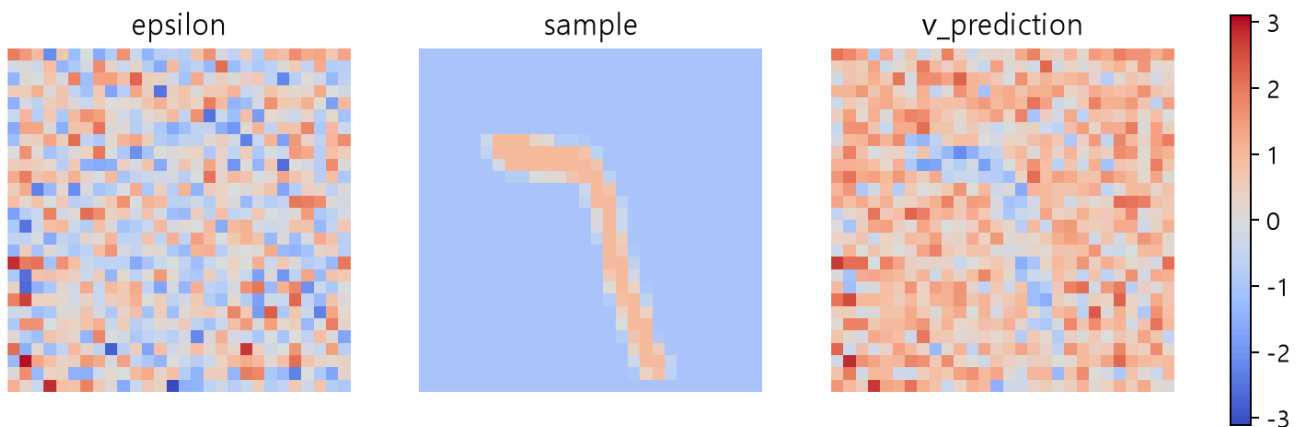
그림 13. 시점49의 실제 원본·잡음으로 만든 정답 target 들이다. 세 배열의 shape은 같지만 의미가 다르다. 같은 대칭 색상 범위를 사용했다. 신경망 세 개를 학습한 성능 비교 그림이 아니다.
