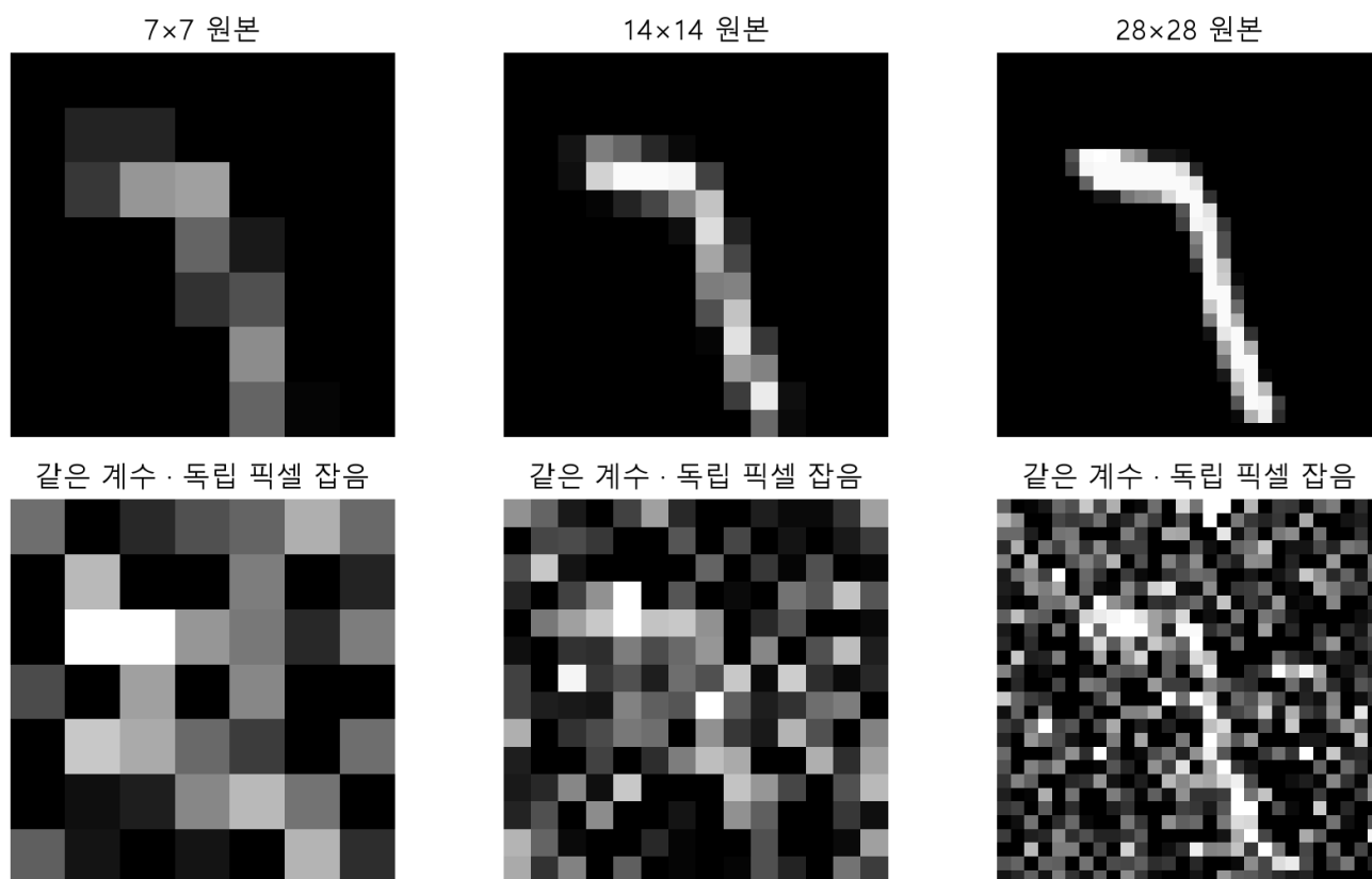
그림 7. 같은 숫자를 area 방식으로 7×7, 14×14, 28×28로 바꾸고 같은 스케줄 시점에 독립 픽셀 잡음을 더했다. 픽셀 수가 달라 잡음 배열 자체가 동일한 것은 아니다. 해상도 외에 모델이나 학습 결과를 비교한 그림도 아니다.
