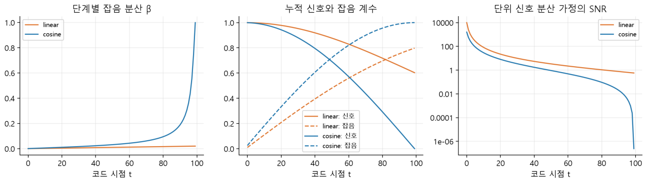
그림 5. 실제 100단계 스케줄의 계산값. 왼쪽은 그 단계의 잡음 분산, 가운데는 누적 신호·잡음 계수, 오른쪽은 단위 신호 분산을 가정한 SNR이다. linear는 beta가 선형이라는 뜻이며, 누적곱이나 신호 계수가 선형이라는 뜻이 아니다. 오른쪽 세로축은 로그 척도다.
