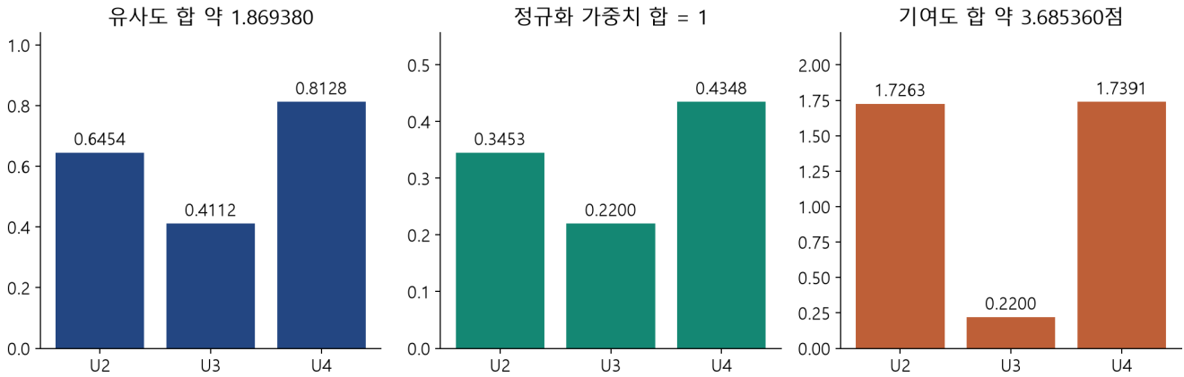
그림 4. 유사도 합은 약 1.869380, 정규화 가중치 합은 1, 평점 기여도 합은 약 3.685360점이다. 세 합 이름과 단위를 구별한다. 그림의 수치는 기존 공개 모델로 직접 계산했다.
