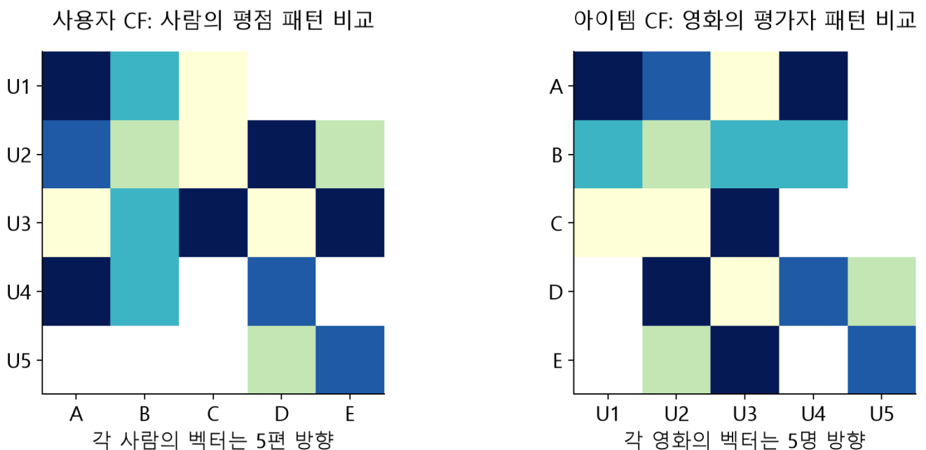
그림 6. 사용자 CF는 비슷한 사람의 D 평점을, 아이템 CF는 D와 비슷한 영화에 U1이 준 평점을 가져온다. 아이템 기반도 줄거리나 장르를 사용하는 콘텐츠 기반 추천과는 다르다.
