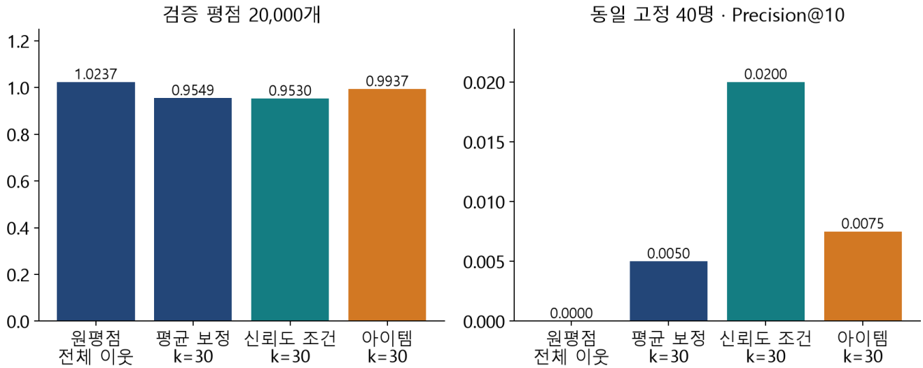
그림 14. 이 실험에서 RMSE가 가장 작은 방법과 카탈로그 노출이 가장 큰 방법은 다르다. 원평점 방식 P@10=0은 고정 40명의 알려진 관련 영화에 적응하지 못했다는 뜻이며, 실제 모든 추천이 싫어하는 영화라는 뜻은 아니다.
