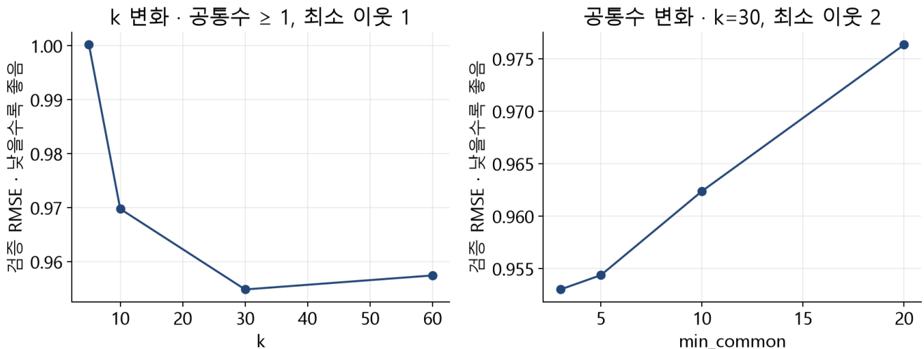
그림 15. 왼쪽은 평균 보정·공통수1·최소1을 고정하고 k를 바꿨다. 오른쪽은 평균 보정·k30·최소2를 고정하고 공통수 하한을 바꿨다. 두 패널 사이에는 최소 이웃 조건이 달라 직접 같은 곡선으로 연결하지 않는다.
