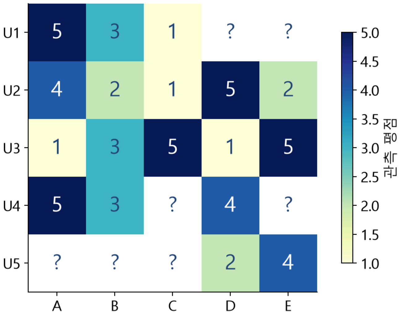
그림 2. U1에게 D 또는 E를 추천하려면 다른 관측에서 근거를 가져와야 한다. 미관측 정답을 만들어 학습 표에 채우지 않는다.
