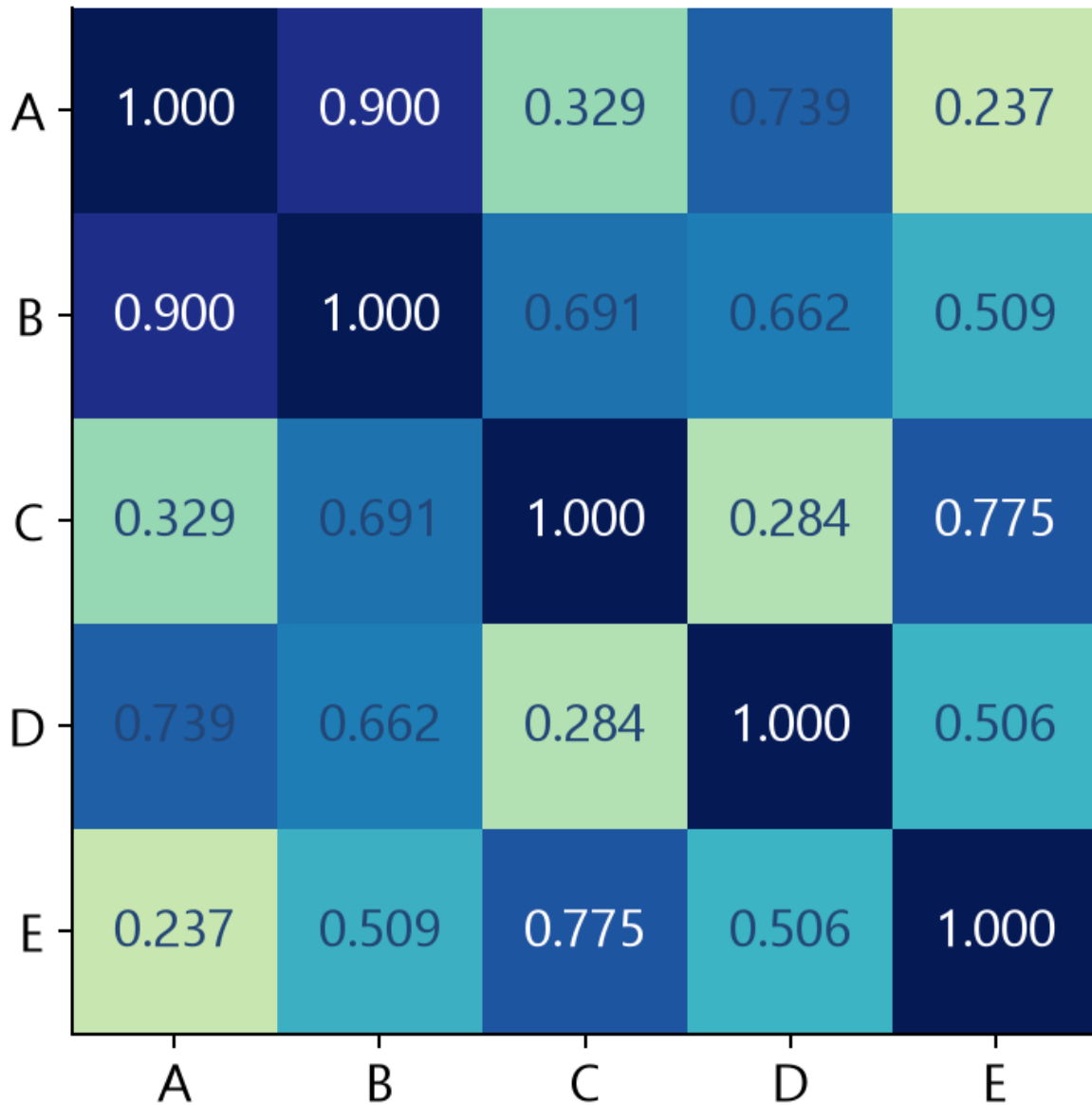
그림 7. D-E의 유사도가 양수여도 U1은 E를 평가하지 않았으므로 U1-D의 근거로 쓸 수 없다. 먼저 U1의 관측 영화 A·B·C로 후보를 제한한 후 그 안에서 상위 k개를 선택한다.
