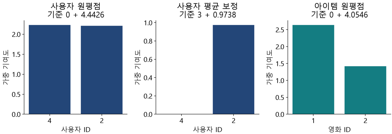
그림 8. 첫 두 그림의 이웃 ID는 사람, 마지막 그림의 ID는 영화다. 막대의 합에 기준 평균을 더하면 각 원예측을 복원할 수 있다.
