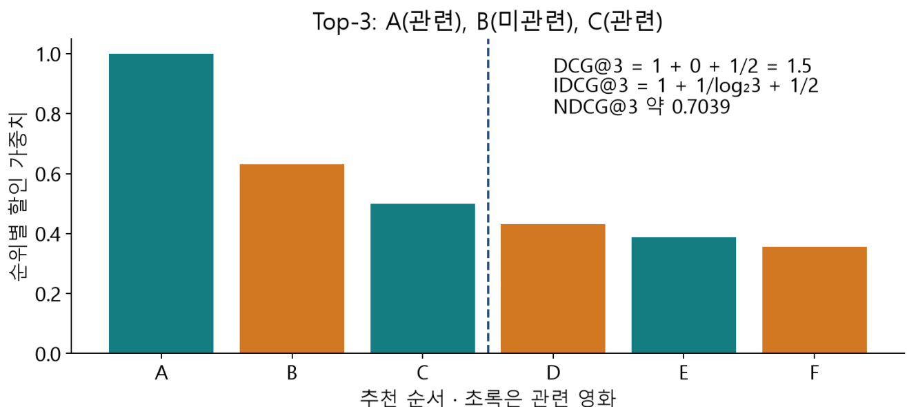
그림 11. 앞의 같은 사례에서 DCG@3=1+0+1/2=1.5다. 관련 영화가 3편이므로 이상적 Top-3은 모두 관련 영화이고, IDCG@3=1+1/log 2 3+1/2≈2.13093이다. NDCG@3≈0.703918이다.
