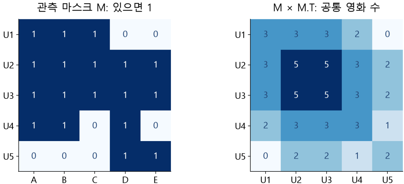
그림 3. U1-U4의 공통 영화는 A·B의 2편, U1-U2와 U1-U3은 A·B·C의 3편이다. 대각선은 자신의 관측 수이며 자기 자신은 이웃에서 제외한다.
