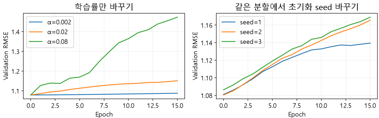
그림 6. 독자 합성 960관측에서 실제 실행한 보강 실험입니다. MovieLens 결과가 아닙니다. 왼쪽은 학습률만 바꾸고, 오른쪽은 같은 분할에서 초기화·방문 순서 seed만 바꿨습니다. seed는 결과를 가장 좋게 만드는 숫자로 골라 발표하기 위한 설정이 아닙니다.
