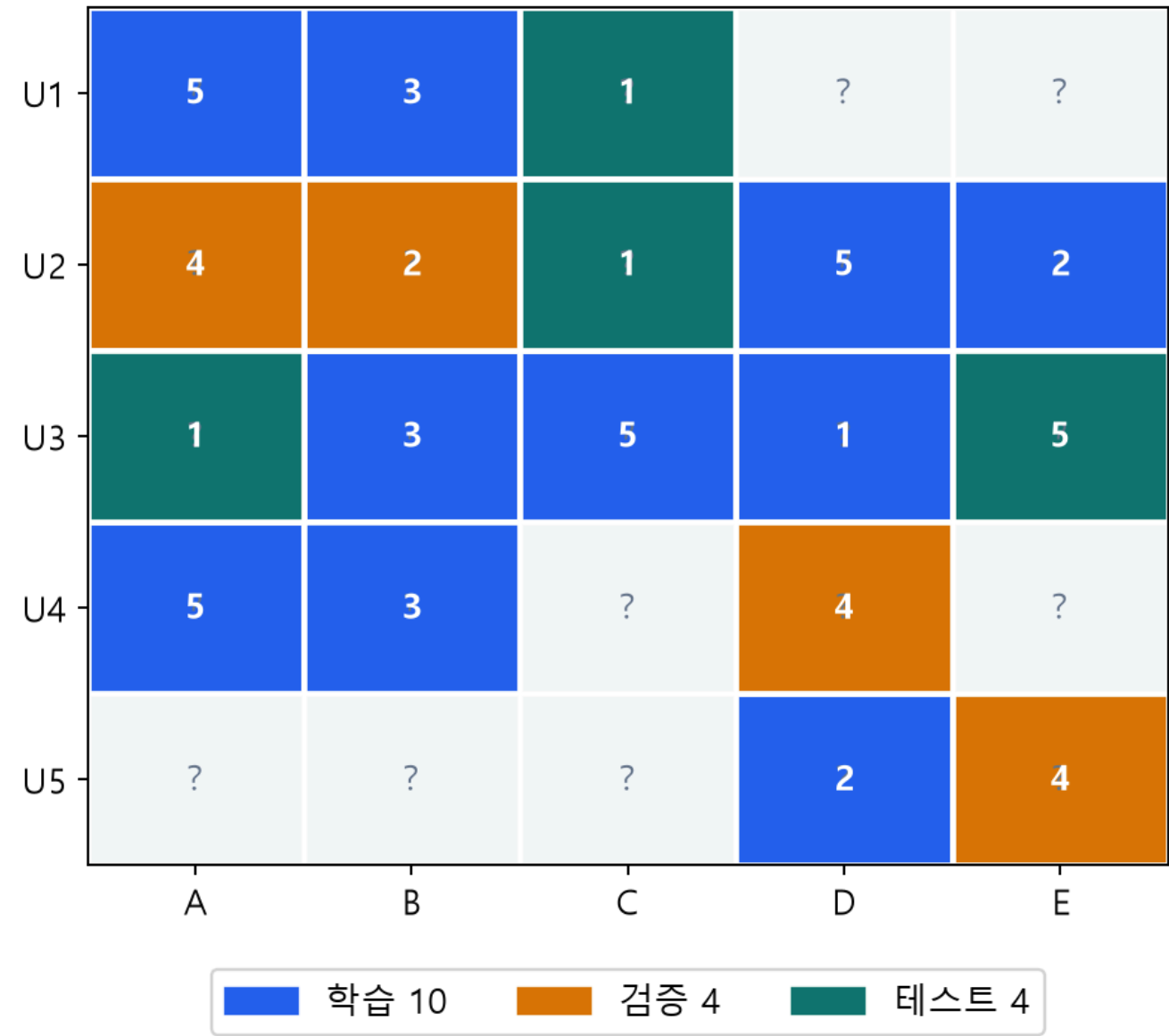
그림 2. W05b와 같은 독자 합성 예제입니다. 실제로 알려진 평점 18개를 10/4/4개로 나누었습니다. 작은 표에 서는 비율을 정수 개수로 반올림합니다. 원래 몰랐던 7칸은 물음표로 남깁니다.
