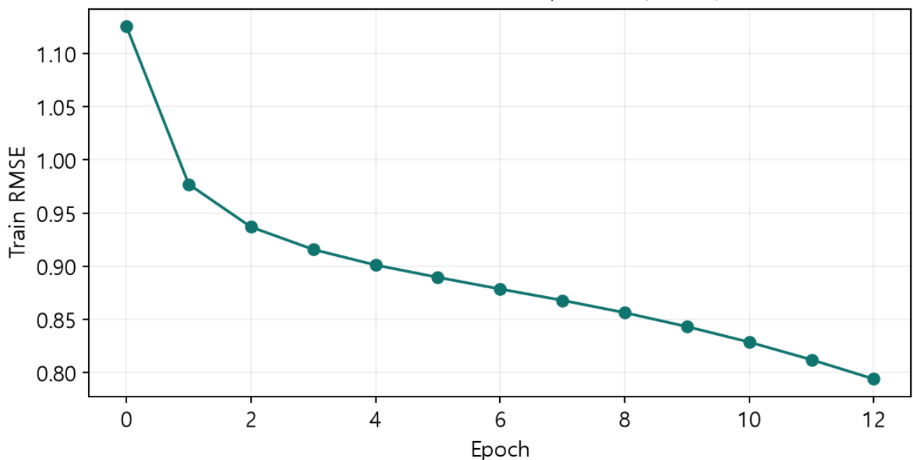
MovieLens 100K 중 고정 20,000관측: 실제 실행
