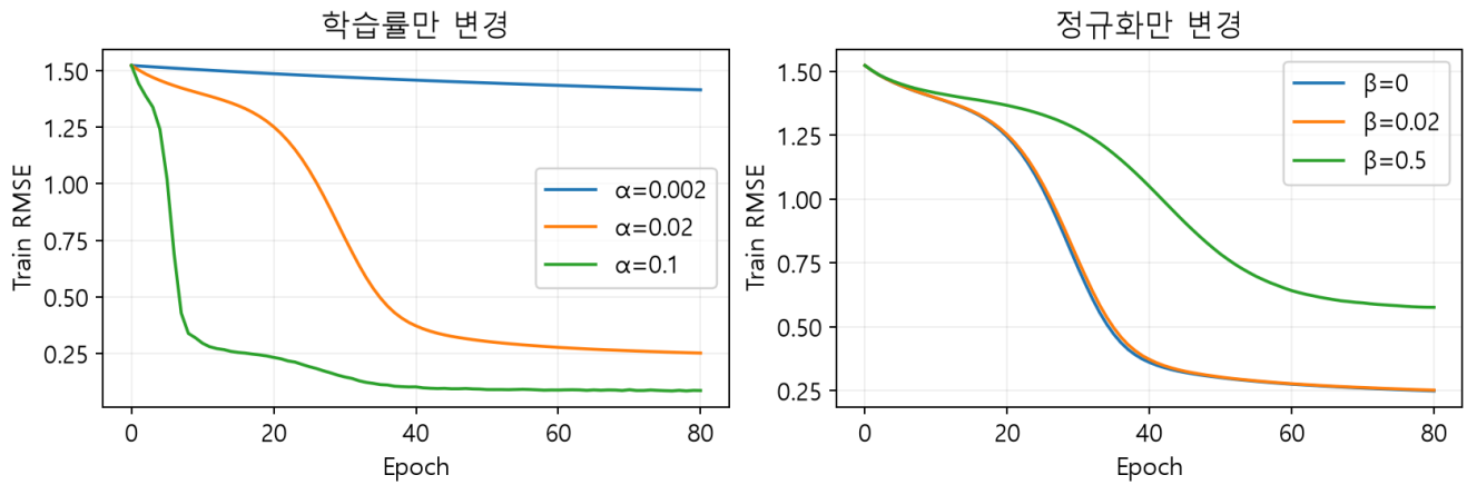
그림 7. 독자 18관측 예제의 실제 실행입니다. 왼쪽은 학습률만, 오른쪽은 정규화만 바꿉니다. “빨리 감소”와 “새로운 데이터에 잘 예측”은 다른 주장입니다. 큰 학습률은 진동이나 발산을 일으킬 수도 있습니다.
