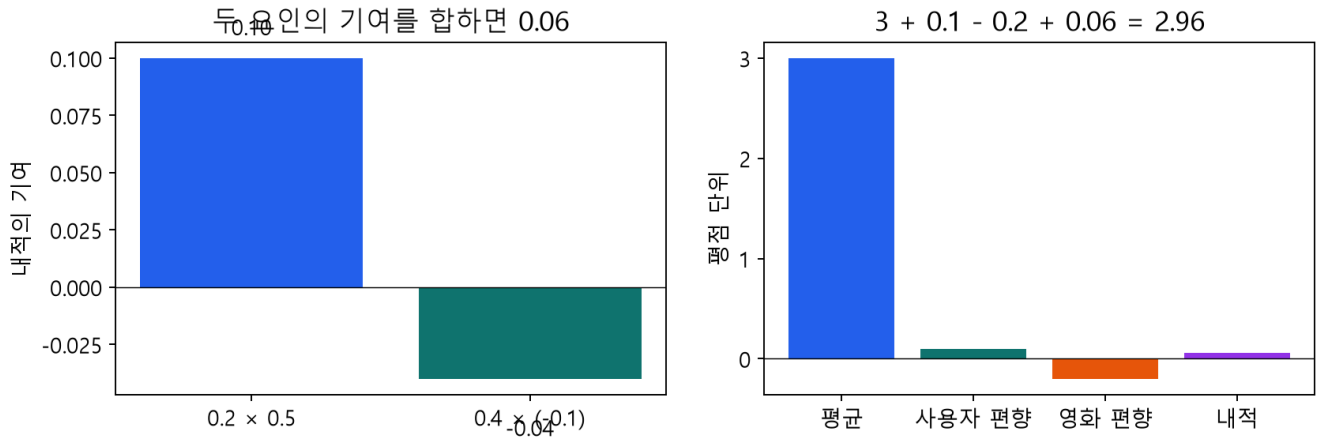
그림 2. 왼쪽 막대는 내적의 두 항입니다. 오른쪽은 뒤에서 추가할 평균·편향을 함께 표시합니다. 음수 좌표를 “음수 평점”이나 “그 장르를 반드시 싫어함”으로 바로 번역하지 않습니다.
