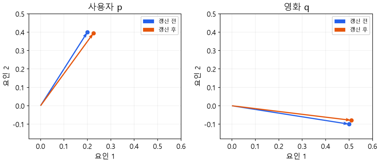
그림 5. 두 벡터가 같은 방향으로 평행 이동하는 것이 아닙니다. 각 벡터가 상대 벡터와 잔차에 따라 이동합니다. 초기값과 새 값을 표·그림·코드에서 대조하세요.
