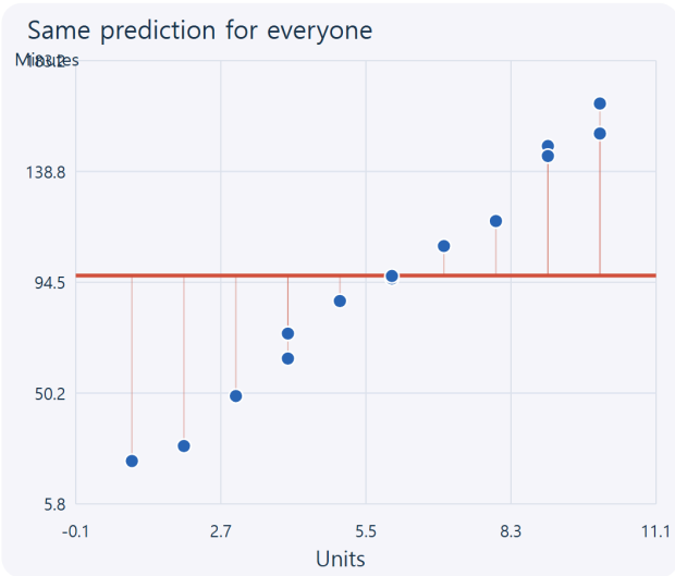
그림 10. 왼쪽은 부품 수를 사용하지 않은 평균 예측이다. 오른쪽은 설명을 위해 제안한 후보 규칙 \hat{Y} = 5 + 15X 다. 이 규칙은 이번 예시에서 비교하기 위해 정한 것이며, 최적이라고 추정한 결과가 아니다. 실제 점과 예측선 사이의 세로 차이에 주목한다.
