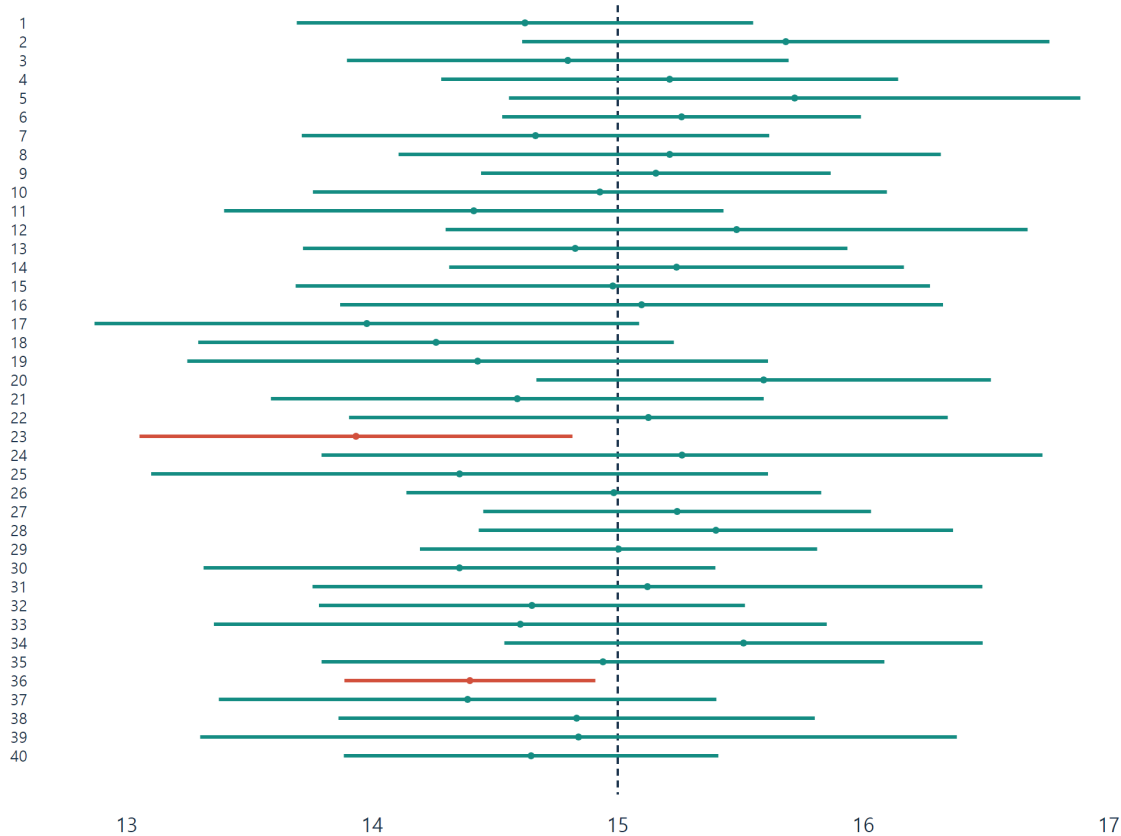
그림 11. 세로 기준선은 참 기울기 15로 고정되어 있다. 각 가로 막대가 새 표본에서 만든 구간이고, 붉은 막대는 참값을 놓친 경우다. 그림의 포괄 수는 실제 시뮬레이션 결과다. 40번처럼 적은 반복에서 정확히 95%가 나와야 하는 것은 아니다.
