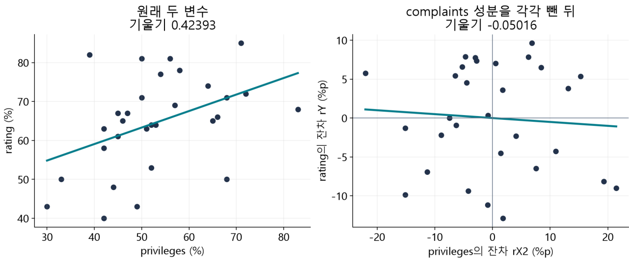
그림 10. 왼쪽은 privileges와 rating의 원래 관계, 오른쪽은 각각에서 complaints와의 선형 관계를 제거한 뒤의 잔차 관계입니다. 오른쪽 기울기는 두 변수 모형의 privileges 계수와 같습니다. 축의 숫자는 원래 긍정 응답 비율이 아니라 각 회귀에서 남은 차이입니다.
