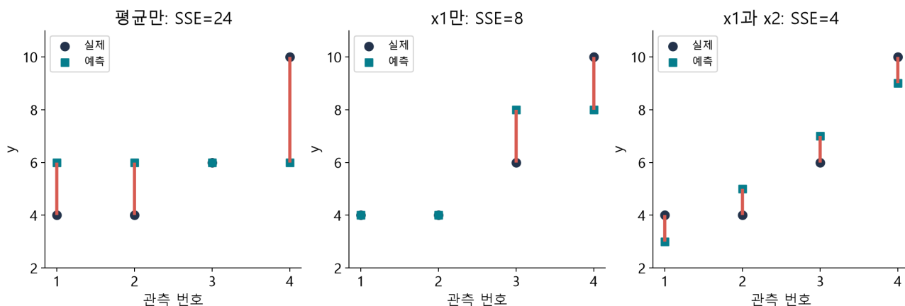
그림 7. 다음 절의 별도 합성 자료에 서로 다른 후보 계수를 적용했습니다. 관측은 고정하고 예측값만 바꿉니다. 왼쪽은 평균 예측, 가운데는 첫 설명변수만 사용한 예측, 오른쪽은 두 변수 최소제곱 예측입니다. 후보별 전체 제곱오차를 비교합니다.
