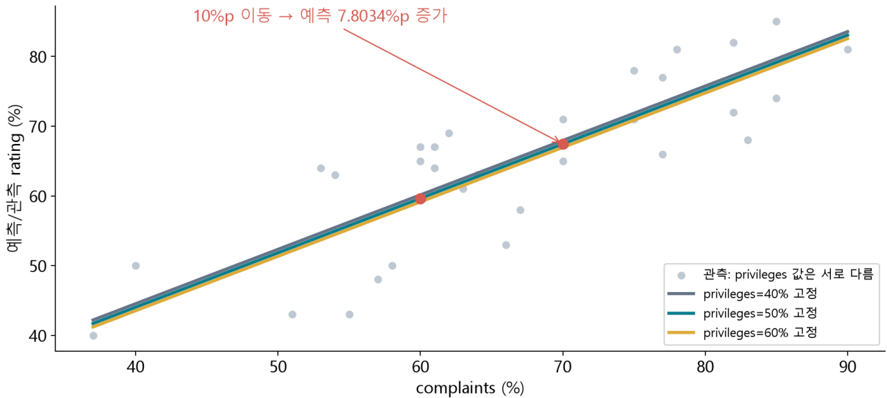
그림 6. 각 선에서는 privileges가 고정되어 있습니다. 선 위에서 오른쪽으로 움직이면 complaints의 계수를 읽습니다. 같은 complaints에서 선 사이를 이동하면 privileges의 계수를 읽습니다. 회색 점들의 privileges는 서로 다르므로 모든 점이 한 단면 직선에 놓일 필요가 없습니다.
