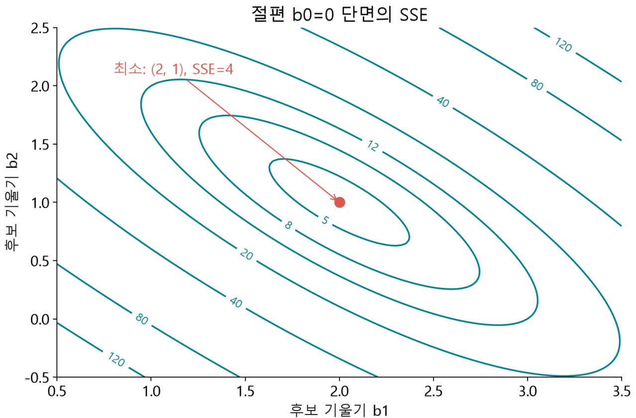
그림 8. 절편을 0으로 고정한 단면에서 (b_1, b_2) = (2, 1) 이 SSE=4 의 최솟값입니다. 점을 따라 계수를 움직이면 손실이 커집니다. 전체 세 계수 최적화의 단면을 보여 주는 그림이지, 절편을 언제나 0으로 두라는 뜻은 아닙니다.
