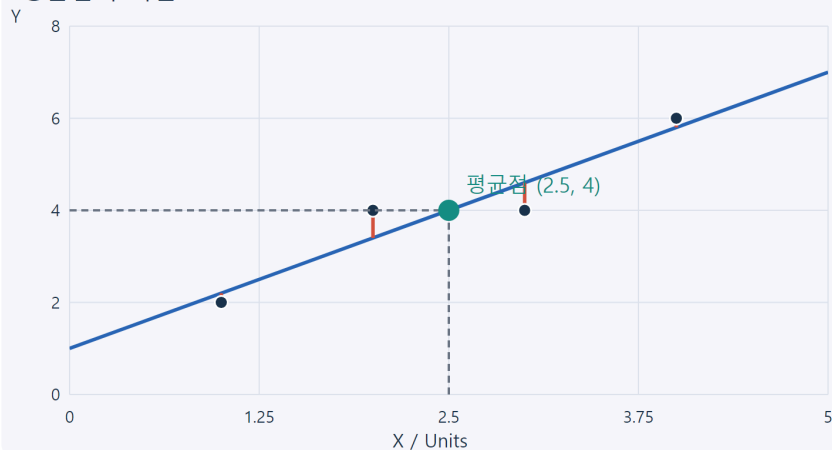
평균점과 직선
