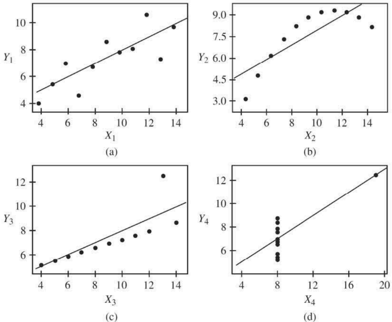
그림 5.1 최소제곱적합선과 산점도: Ancombe's Quartet
