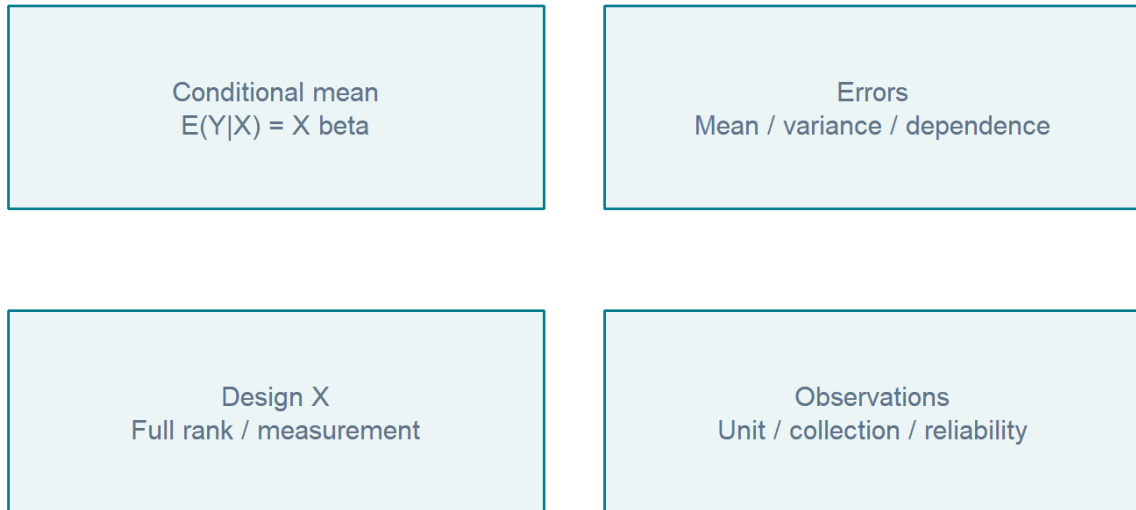
그림 A2. 왼쪽 위는 평균을 설명하는 식, 오른쪽 위는 그 평균 주위의 오차, 왼쪽 아래는 설명변수 정보, 오른쪽 아래는 자료가 만들어진 과정을 뜻합니다. 서로 다른 상자에 대한 주장을 혼합하지 마세요.
