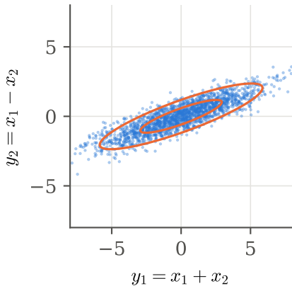
Y = AX : ACA^T
