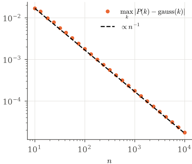
(b) de Moivre--Laplace error, p = 0.3
